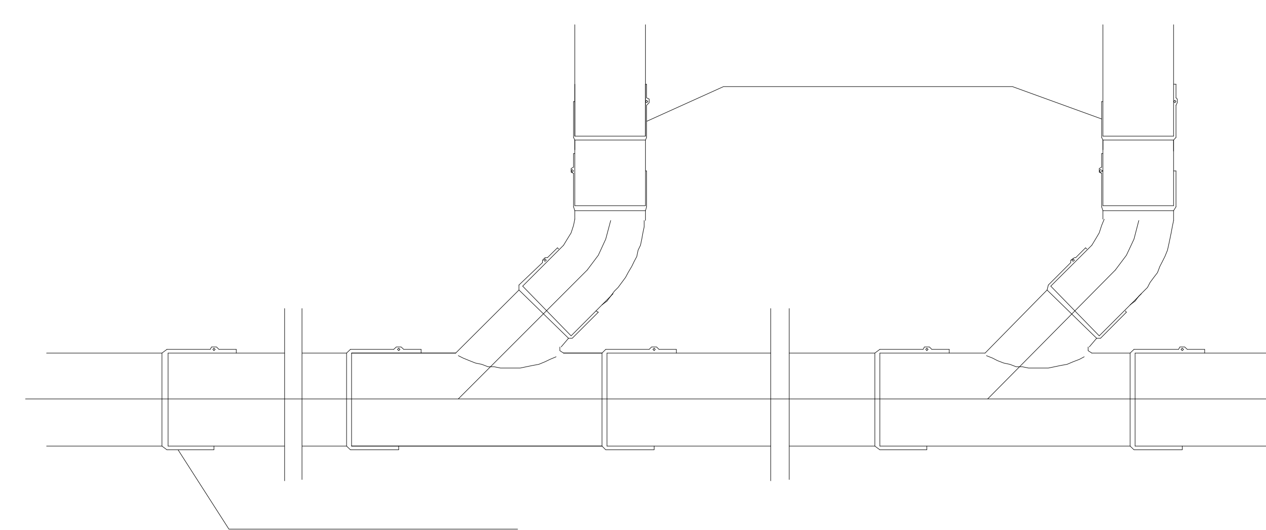
SKEMA E LIDHJES SE KOLONAVE ME KOLEKTORET HORIZONTALE TE SHKARKIMIT
