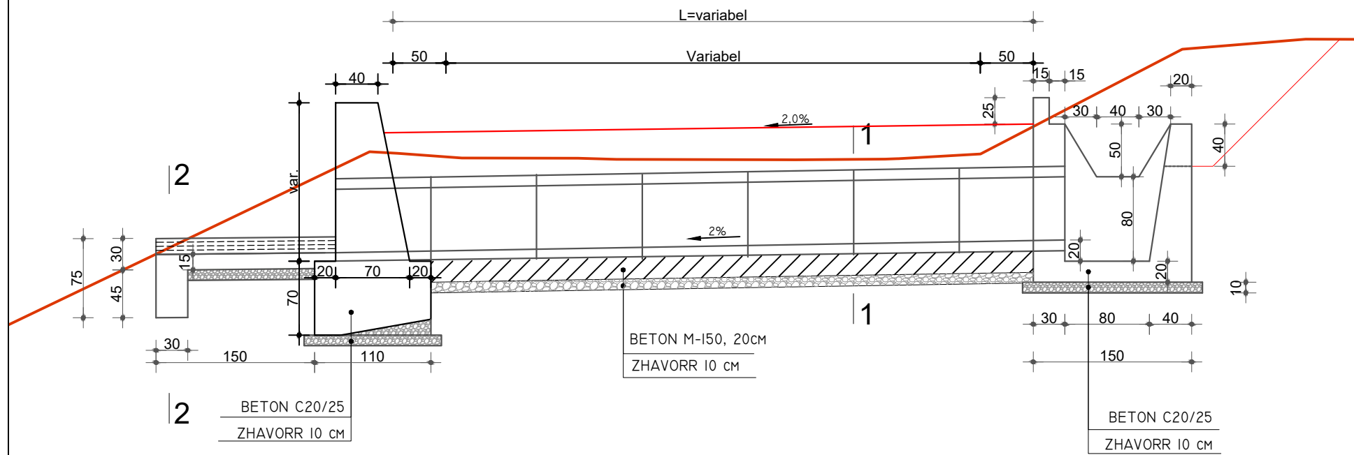
Prerje 1-1
