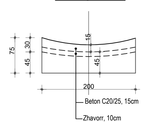
Prerje 2-2
