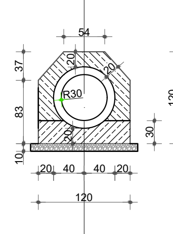
Prerje 1-1
