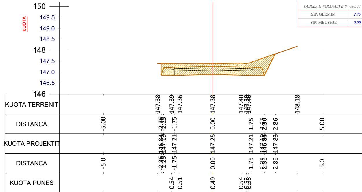
CS - 5 PROG - 0+080.0
