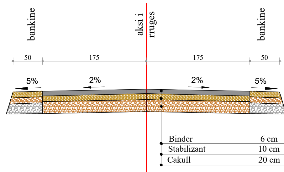
PROFILI TIP 1 PG CS-0 - CS - 63
