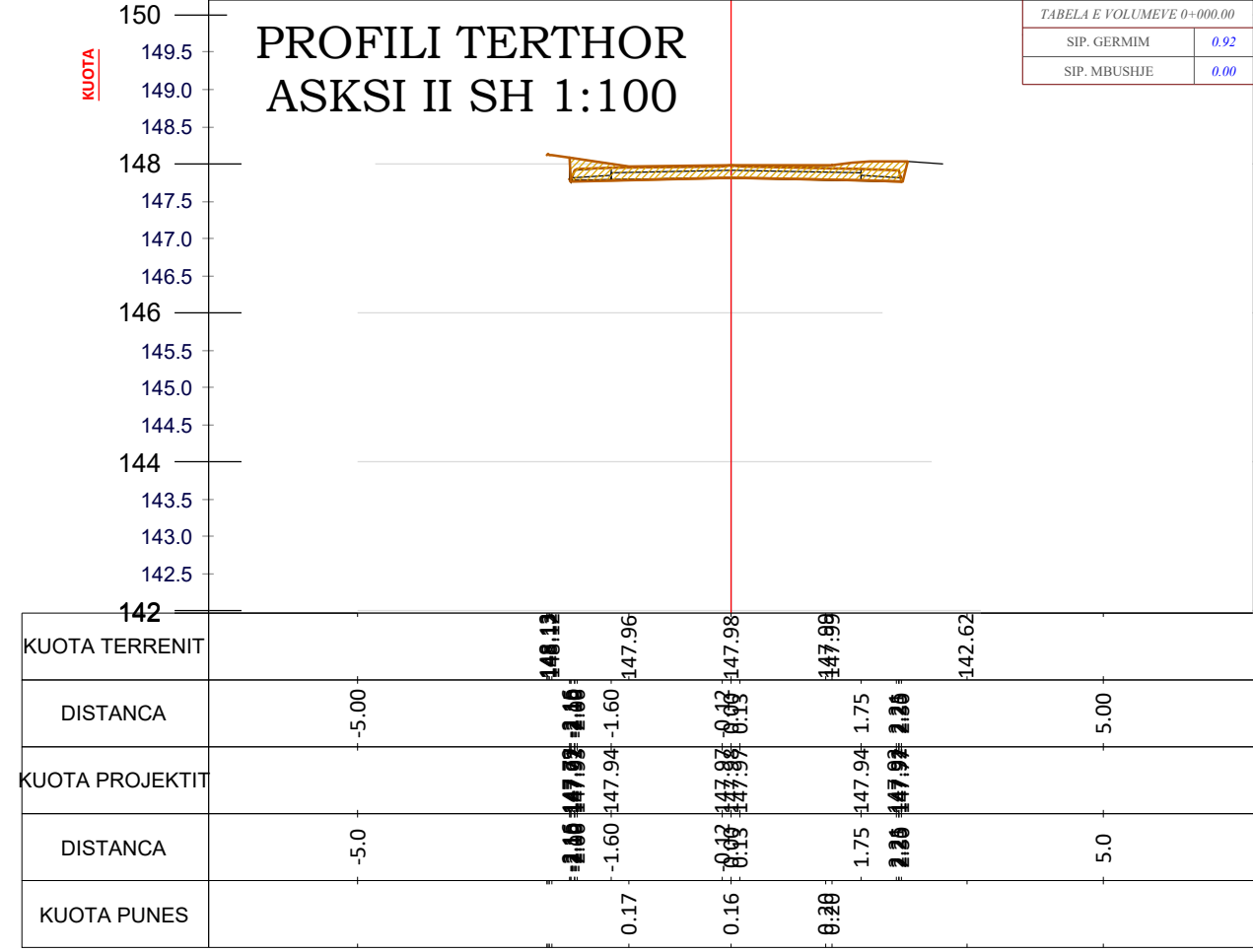
CS - 10 PROG - 0+180.0
