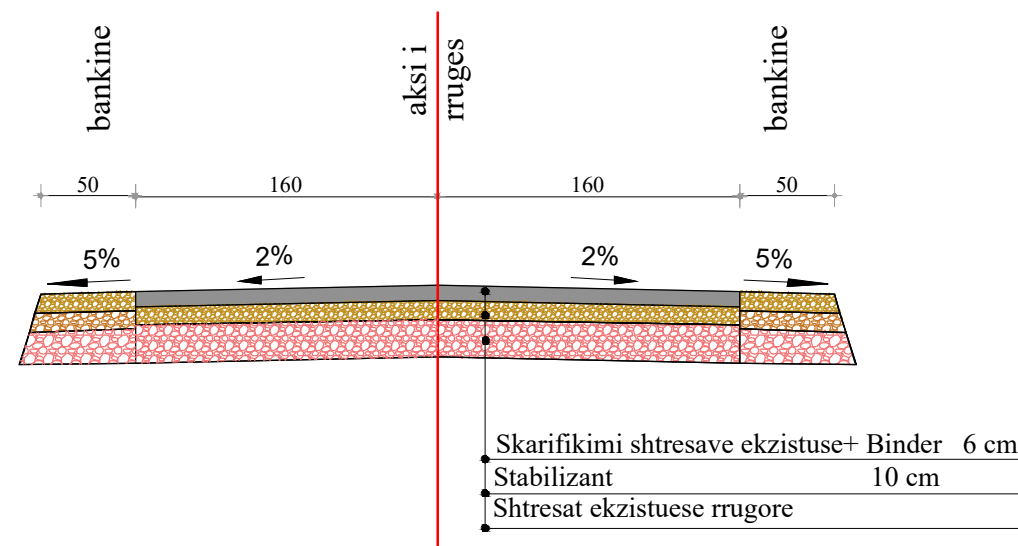
PROFILI TIP 2 NE AKSIN 2 PG CS-0 - CS 0+10 m : PG CS-3+10.5 m - CS 7+2.5 m : PG CS-9+18 m- CS-11+7 m
