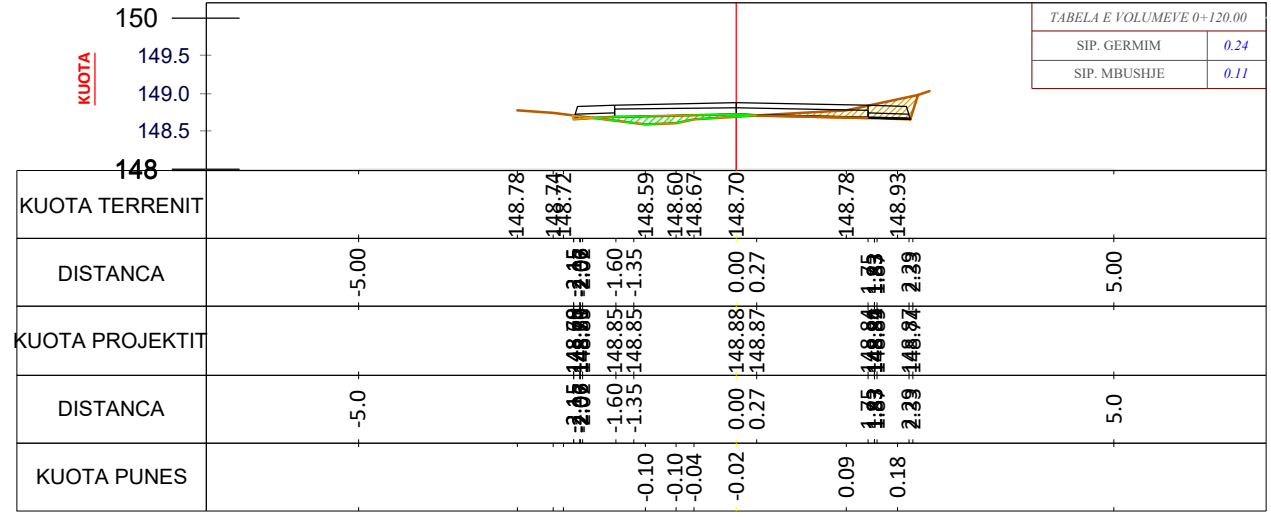
CS - 7 PROG - 0+120.0
