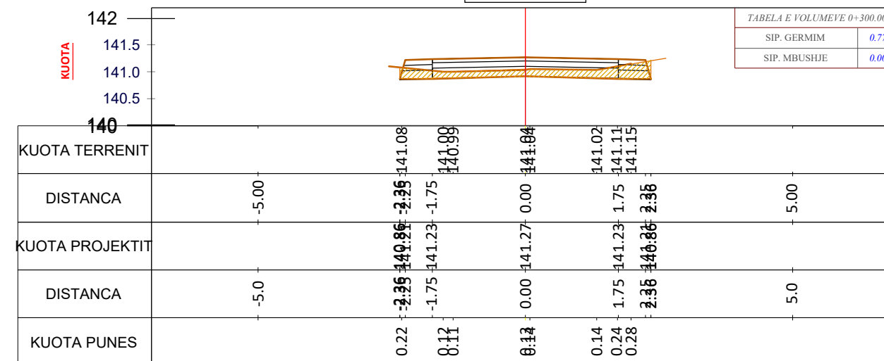
CS - 16 PROG - 0+300.0
