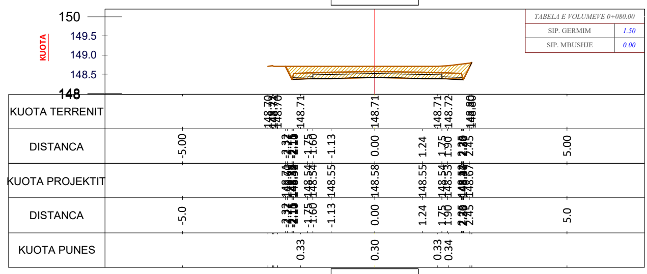
CS - 6 PROG - 0+100.0
