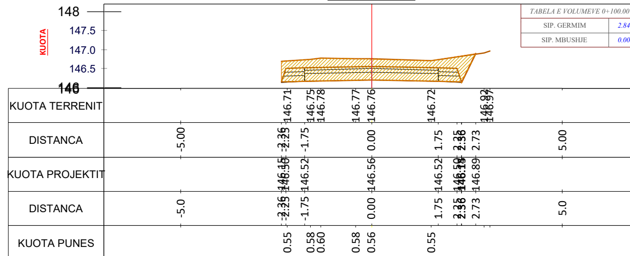
CS - 6 PROG - 0+100.0
