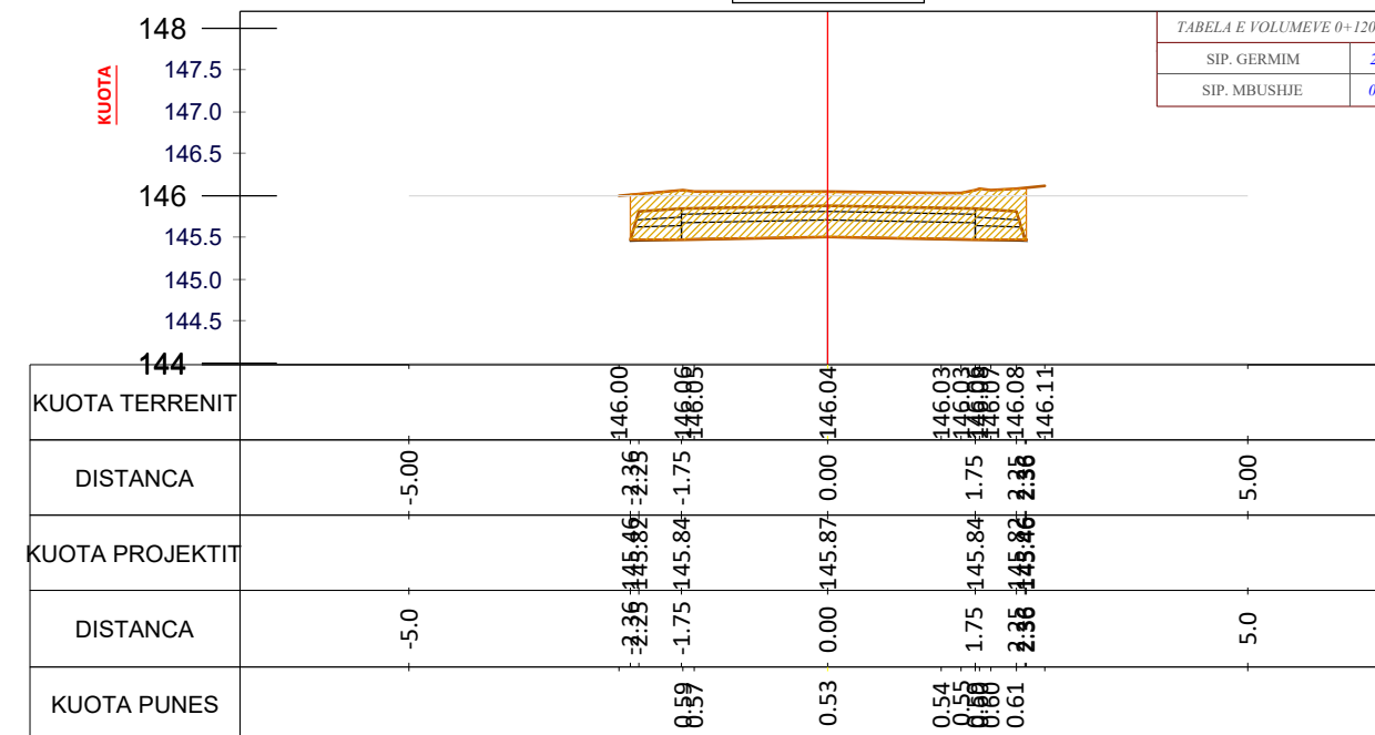
CS - 7 PROG - 0+120.0
