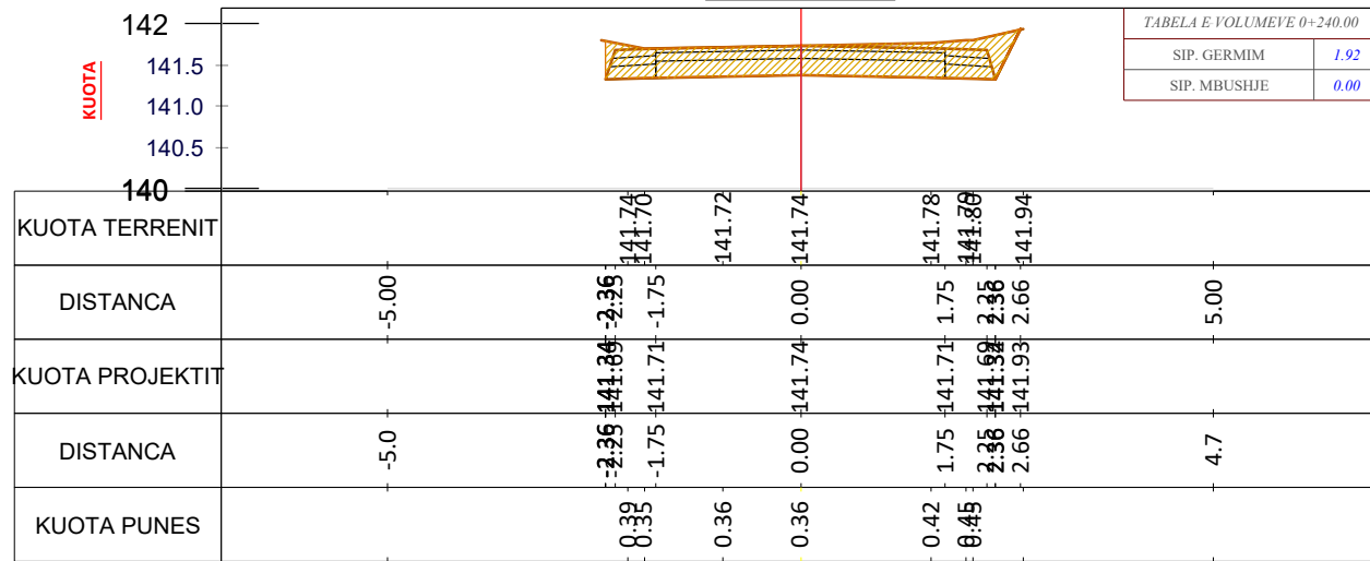
CS - 13 PROG - 0+240.0
