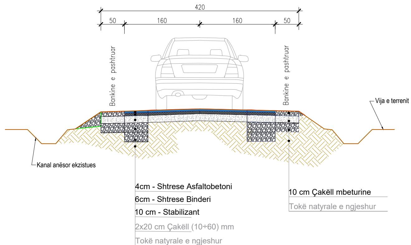
SEKSIONI TERTHOR TIP (ASFALT I RI) PK.2-PK.3, PK.4-PK.5, PK.6-PK.7
