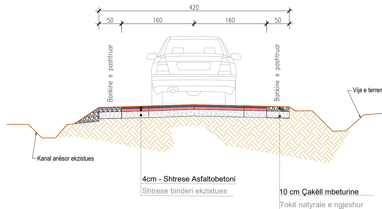
SEKSIONI TERTHOT TIP 2 (RIVESHJE) PK.1-PK.2, PK.3-PK.4, PK.5-PK.6, PK.7-PK.8
