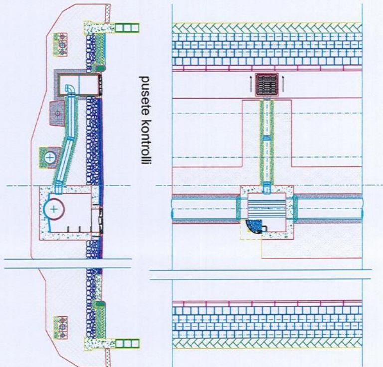
Planimetri dhe seksione rugeore tip
