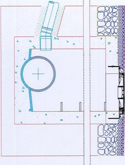
Puste kontrolli ne linje - derdhje nga kapaku tub shkarkimi betoni Ø 500
