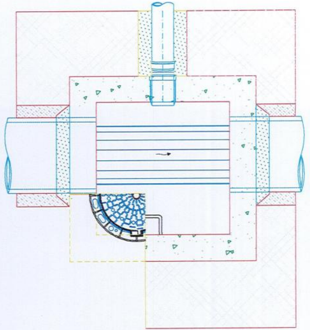
Puste kontrolli ne linje - derdhje nga kapaku tub shkarkimi betoni Ø 500
