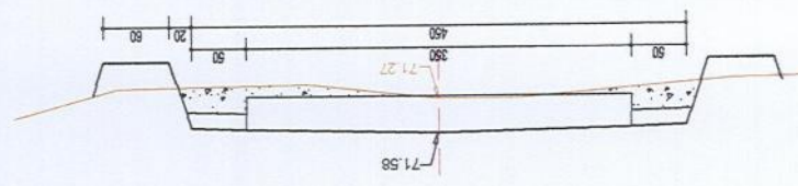
Pr. 8 Pr = 186.0 m
