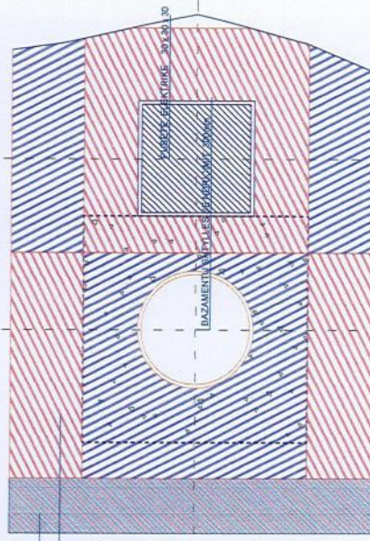
DETAJI -B3 SHKALLA 1:10
