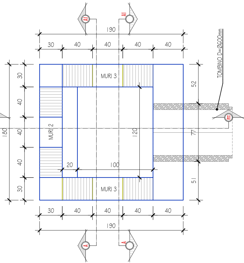
Plani i Pusetës, Sh. 1:30
