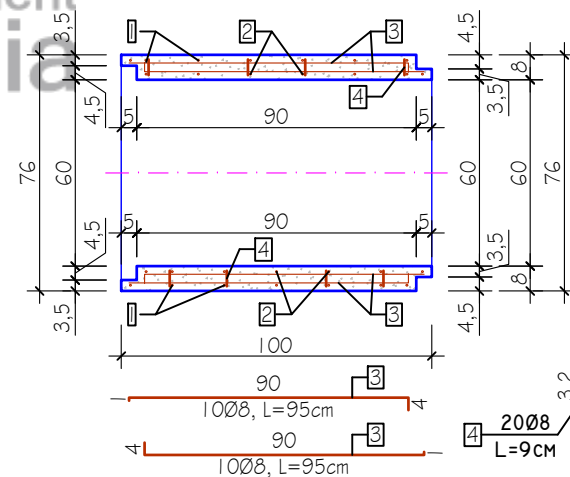
ARMATURA SPIRALE PËR D=60cm
