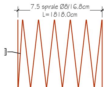
ARMATURA SPIRALE PËR D=60cm
