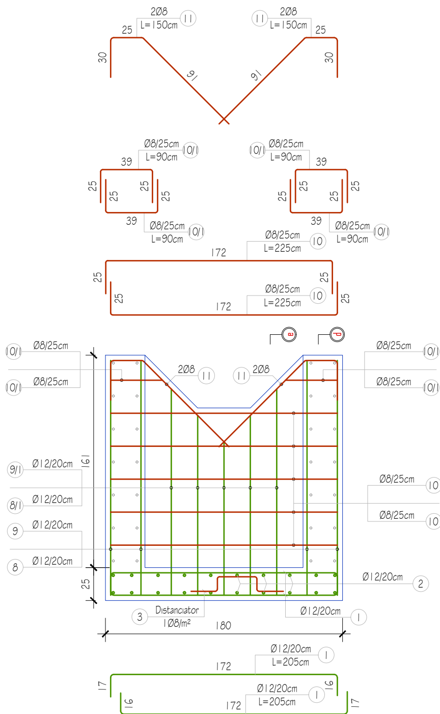
Armimi i Munt 2 të Pusetës, Sh. 1:30
