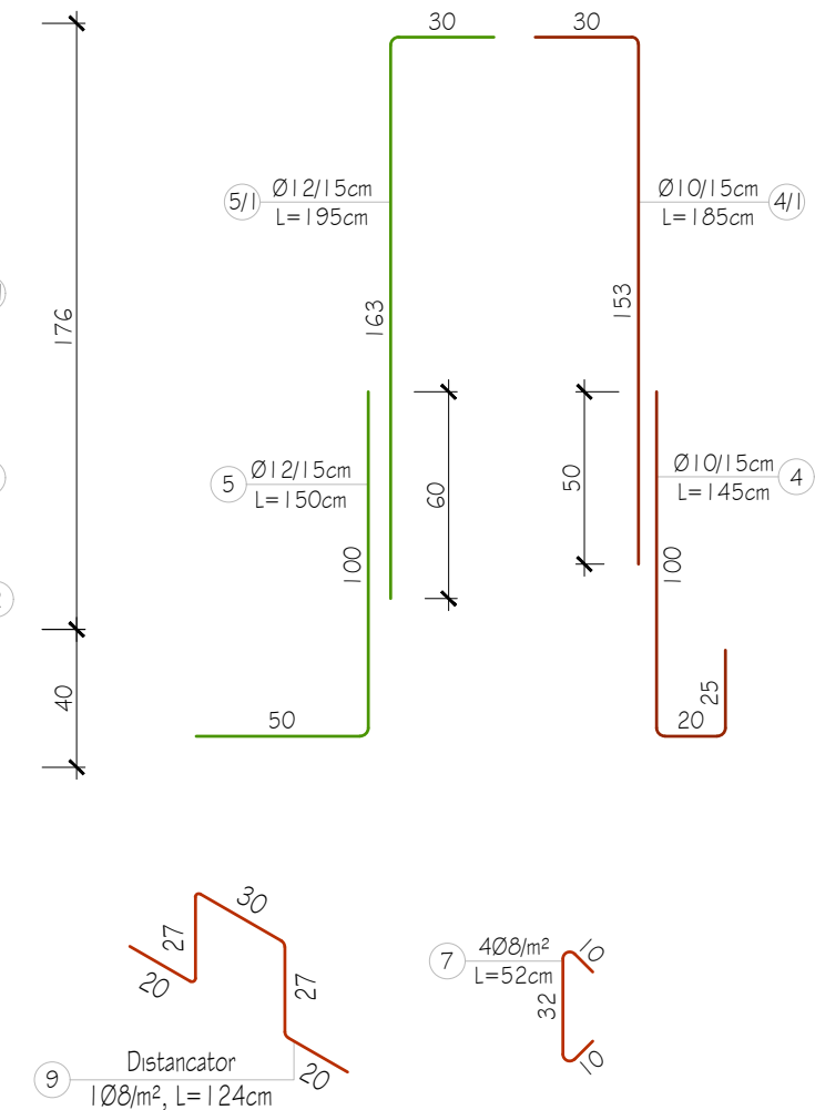
Prerja 1-1 Armimi i munt b/a të portalit të drejtë të tombinos Ø600mm, Sh. 1:25
