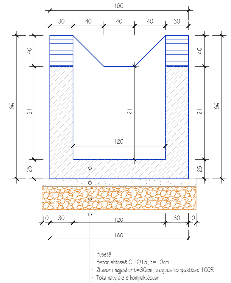
Prerja 2-2 e Pusetës, Sh. 1:30
