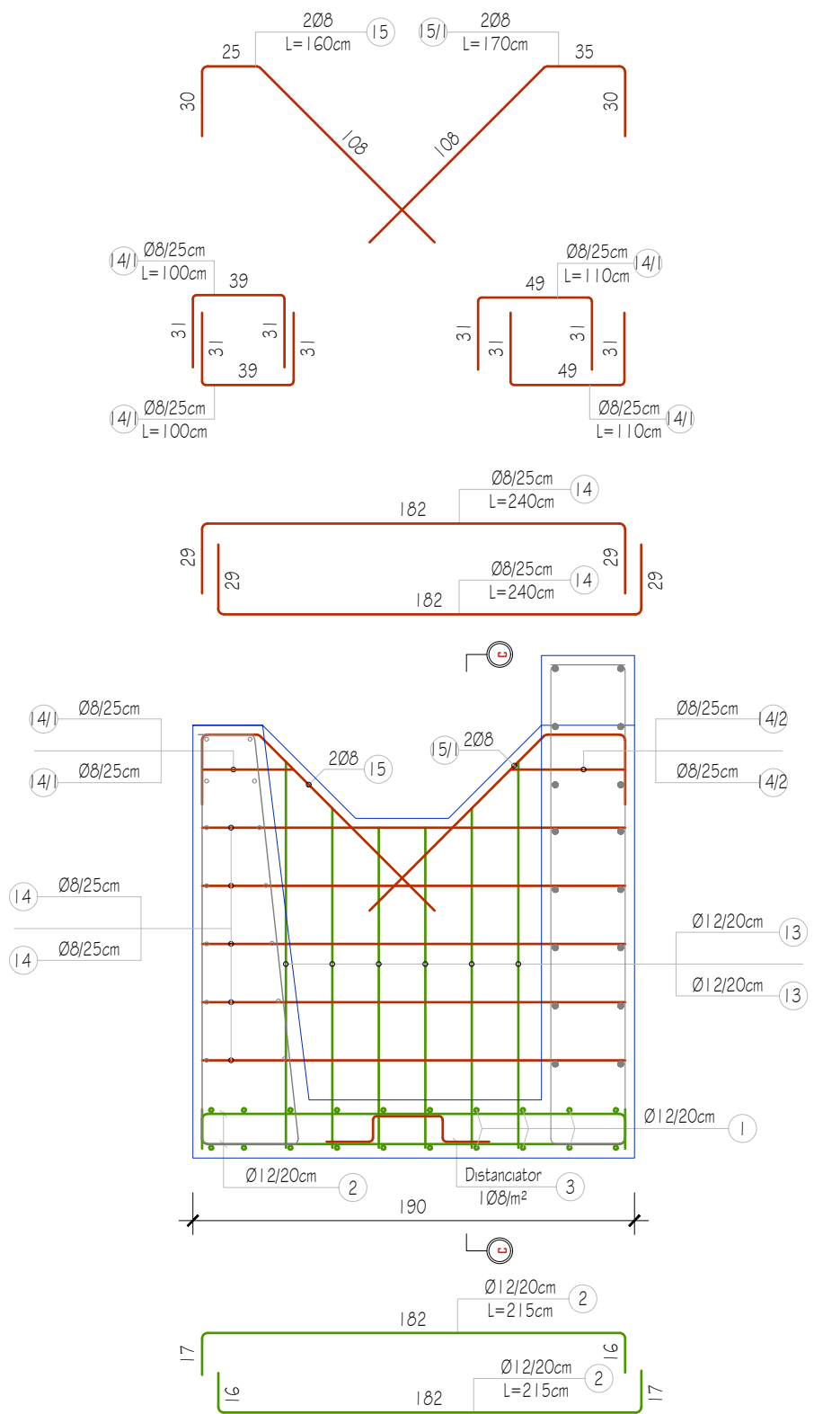
Armimi i Murit 3 të Pusetës, Sh. 1:30
