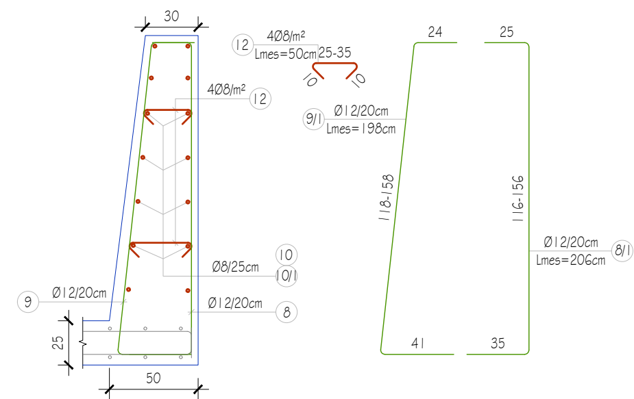
Prerja e-e, Armimi i Munt 2 të Pusetës, Sh. 1:30
