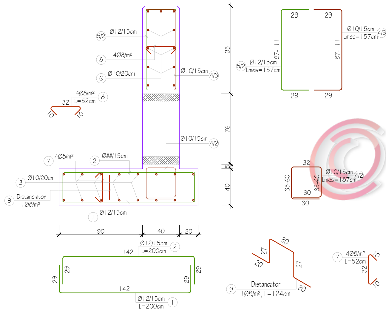
Prerja 1-1 Armimi i murit b/a të portalit të drejtë të tombinos Ø600mm, Sh. 1:25
