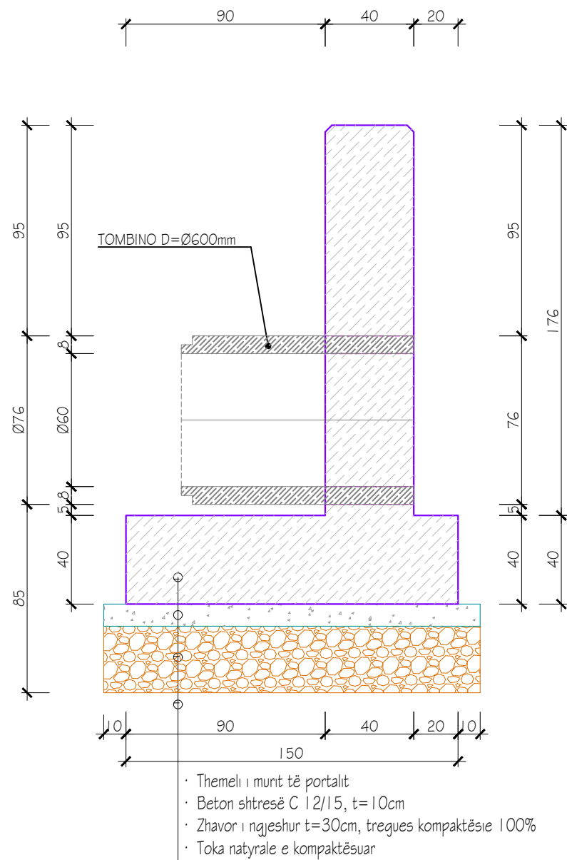
Prerja 1-1 e Munt b/a të portalit të drejtë të tombinos Ø600mm, Sh. 1:25
