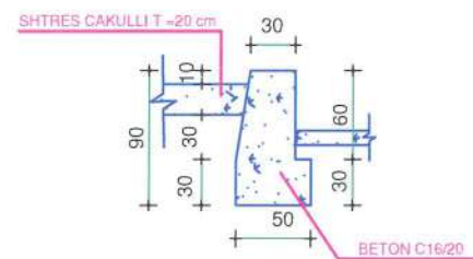
PRERJA A-A SH. 1:50
