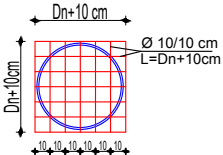
DETAJ I ZGARES HYRJE-DALJE SHk. -1 : 50
