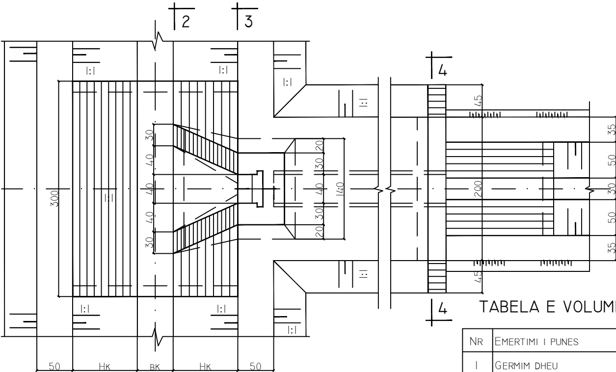
PRERJA 6 - 6
