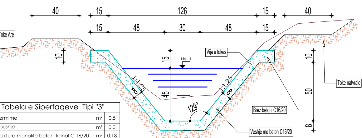
Kanal Primar Tipi "3" Shk. 1 : 20
