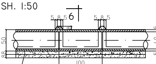
PRERJA 7 - 7
