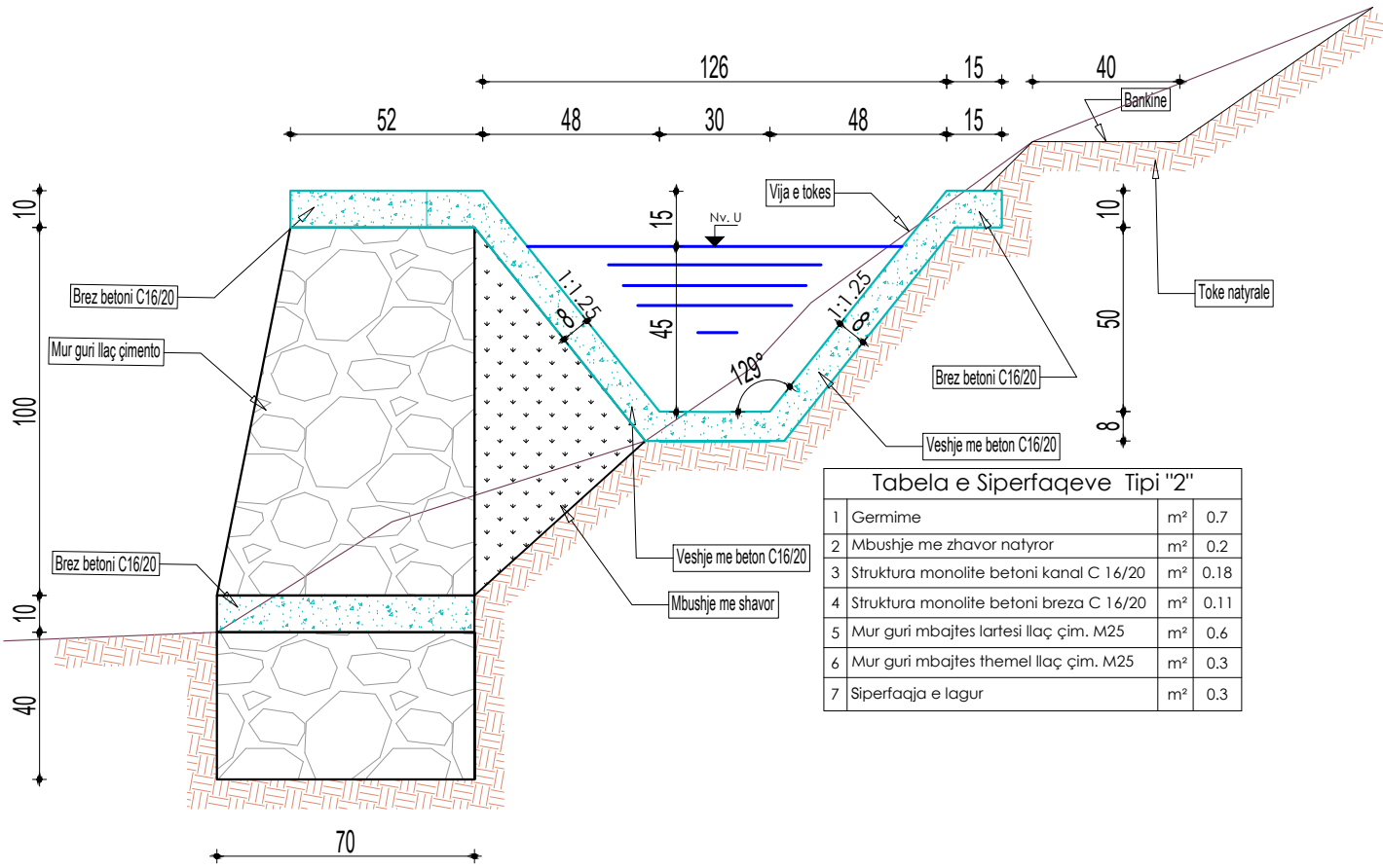
Kanal Primar Tipi "2" (me mur mbajtes) Shk. 1 : 20
