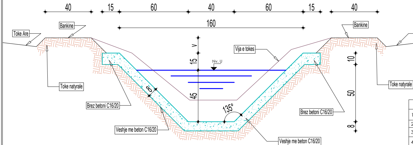
Kanal Primar [ne toke are] Tipi "1" Shk. 1 : 20
