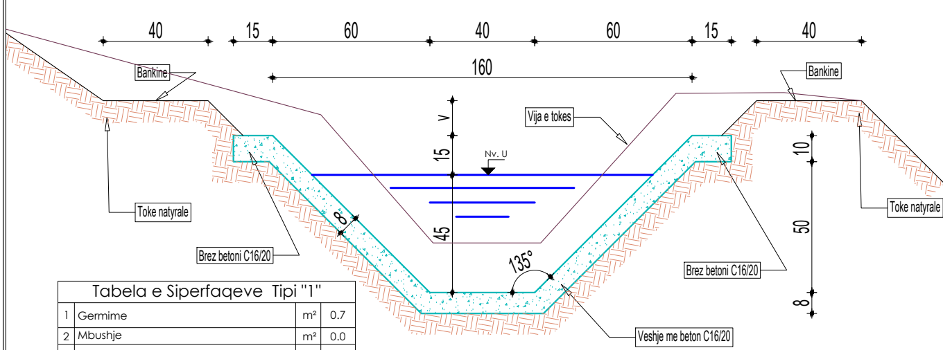
Kanal Primar [ne shpat te pjeret] Tipi "1" Shk. 1 : 20
