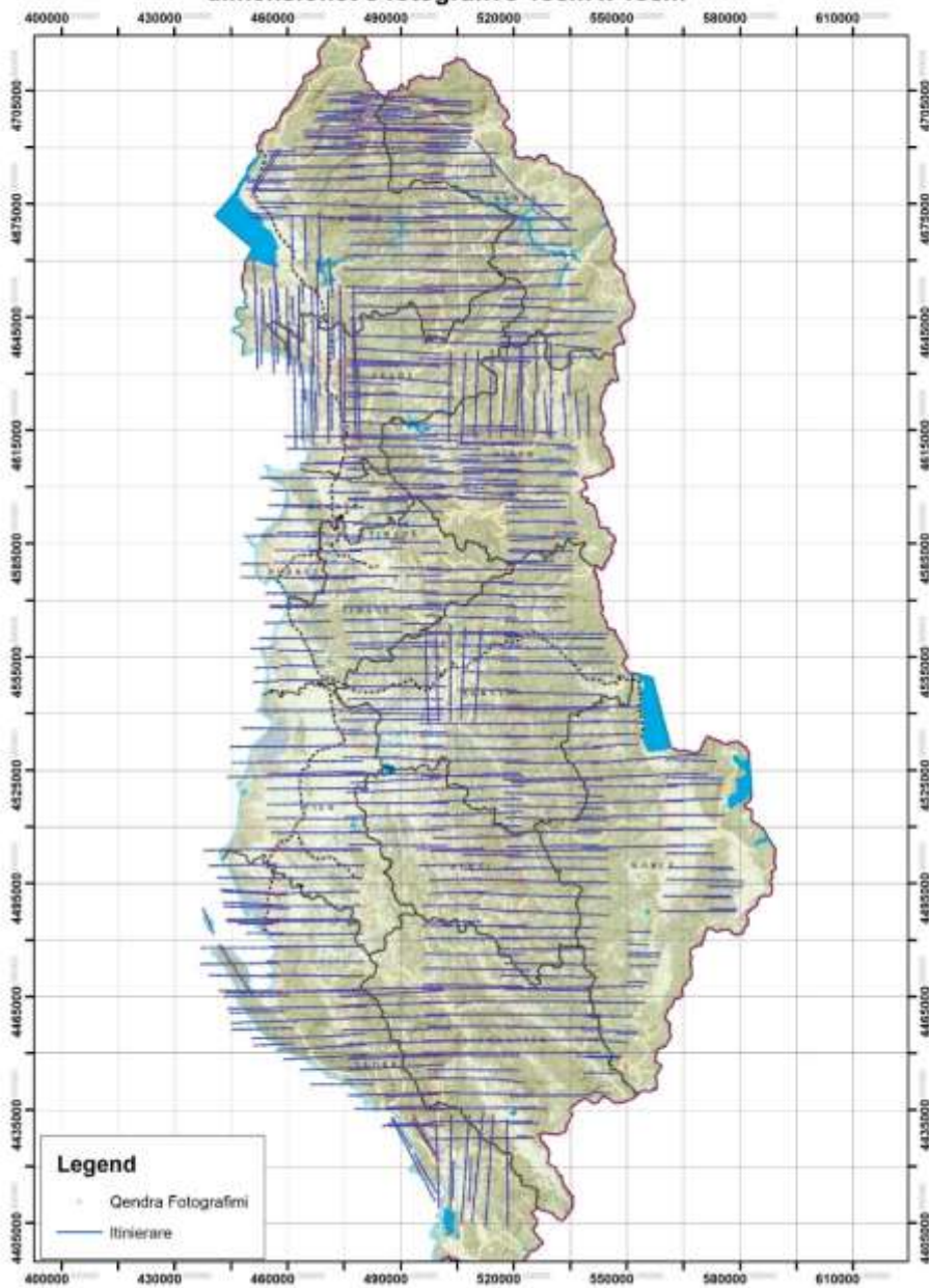
Skema fotografim 1957, shkalla 1:25000, dimensionet e fotografive 18cm x 18cm
