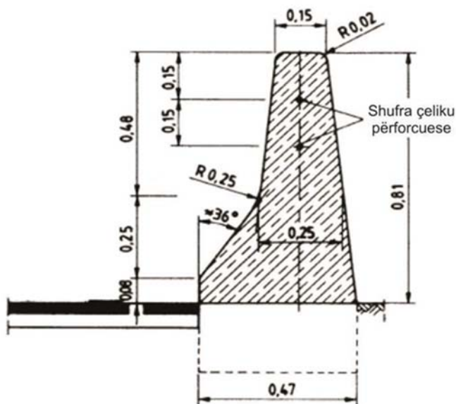
Barriera sigurie prej betoni me një faqe BBS
