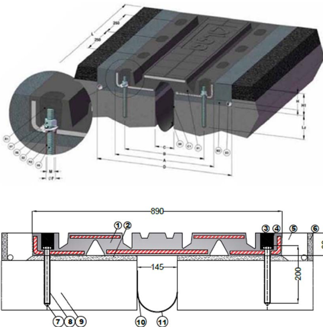
Detaj Teknik – Fuga 890 ÷ 900 mm
