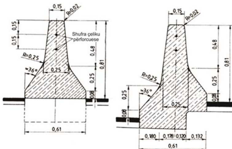
Barrierë sigurie prej betoni me dy faqe
