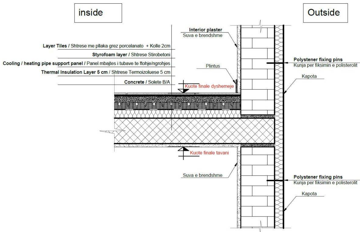
Fig. 19 – detaje te montimit te sistemit KAPOT
