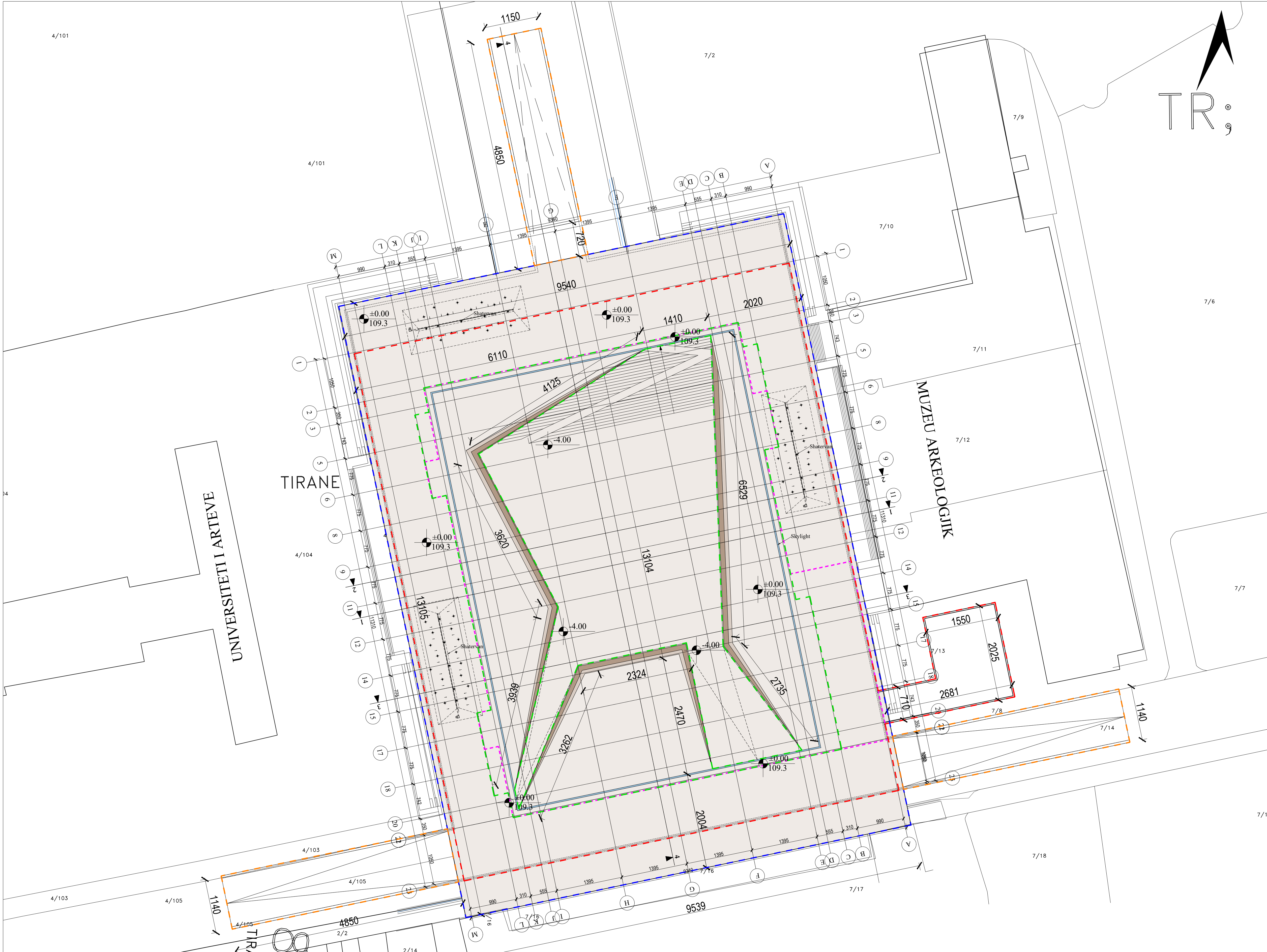
PLANI I VENDOSJES SË STRUKTURËS SHK. 1: 400
