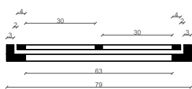
PRERJE B -- B
