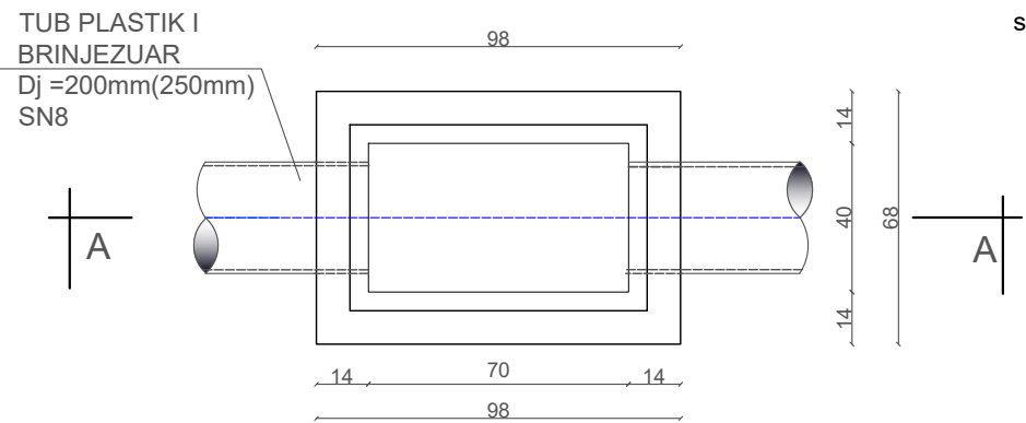
PLANIMETRIA SHK.1: 20
