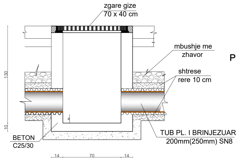
PRERJE A - A SHK.1: 20
