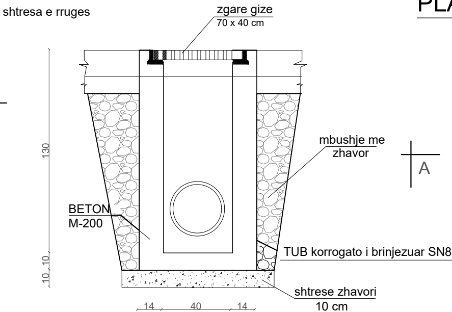
PRERJE B - B SHK.1:20
