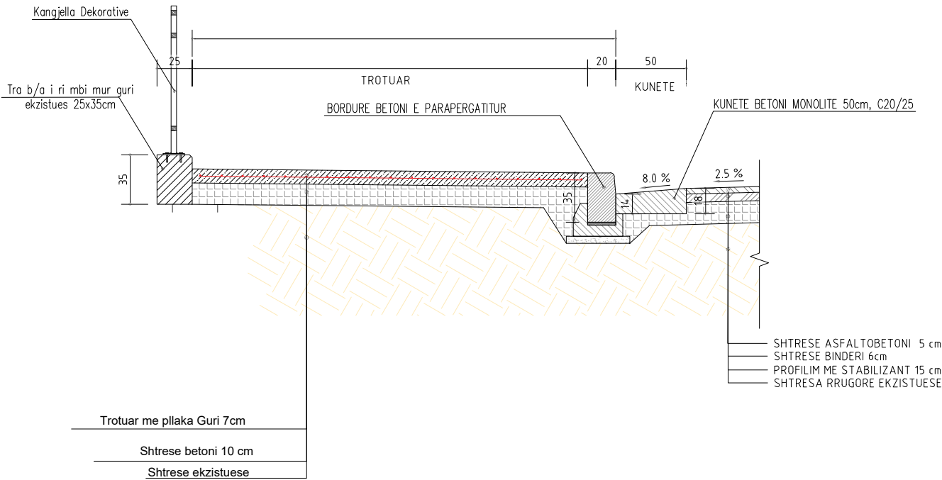
DETAJI I KUNETES, BORDURES DHE TROTUARIT SHKALLA A1- 1:20
