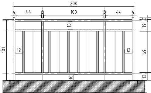
DETAJI I KANGJELLES METALIKE SHKALLA A1- 1:20
