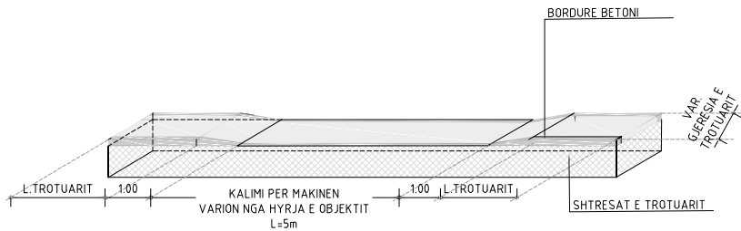
DETAJE I ULJES SE TROTUARIT NE HYRJE-DALJE
