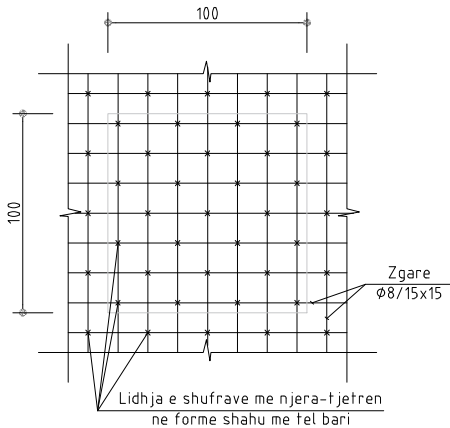
DETAJE TE ELEMENTEVE RRUGOR SHKALLA 1:100
