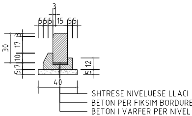
DETAJE DHE DIMENSIONE TE BORDURAVE SHKALLA A1- 1:20
