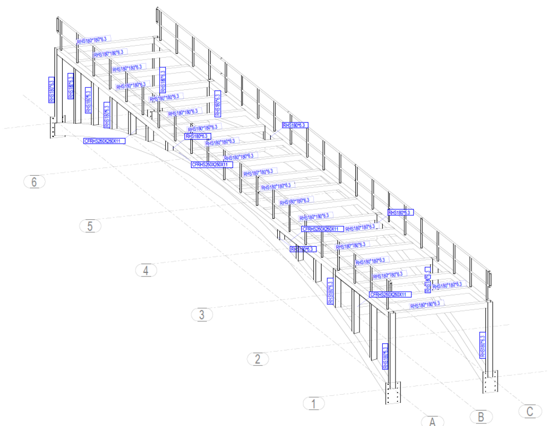
Paraqitje 3d e konstruksionit metalik te Urave tip te kembesoreve
