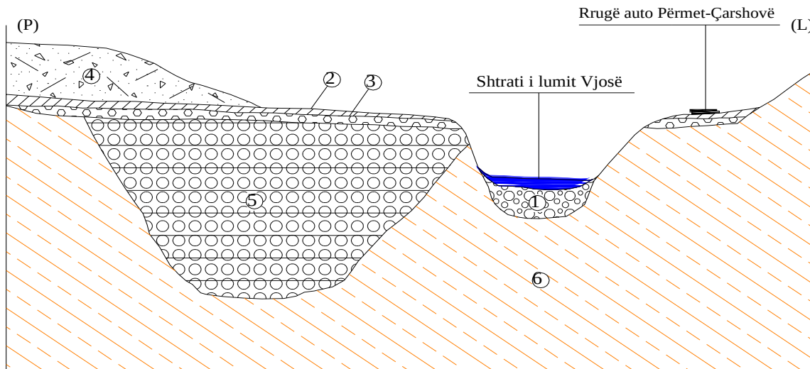
fig.2 PRERJE PERFAQESUESE GJEOLIGO - INXHINIERIKE E BAZES SE LUGINES TE LUMIT VJOSE PRANE MALIT TE BARDHE.
