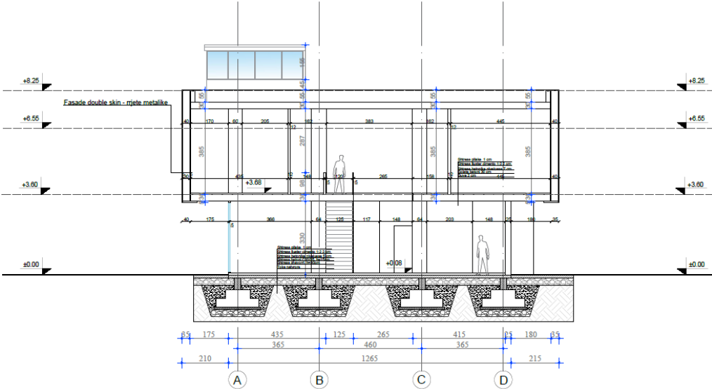
Prerja B-B
