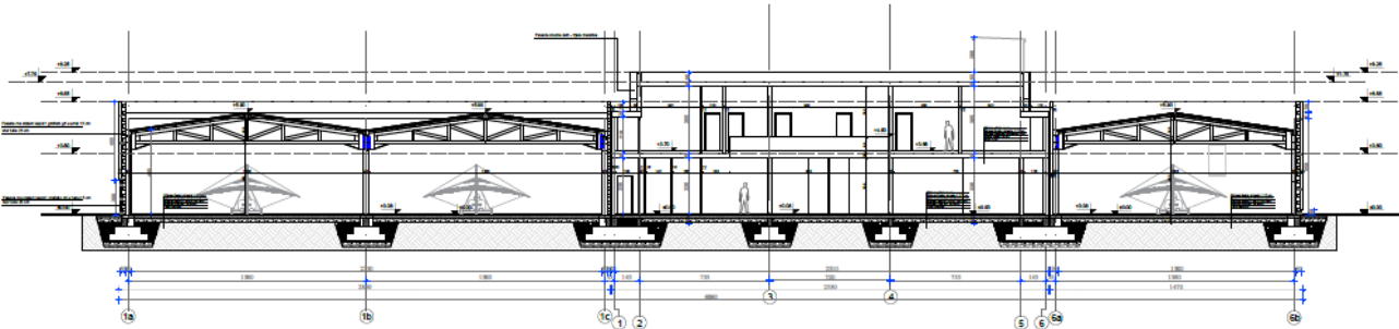
Prerja B-B
