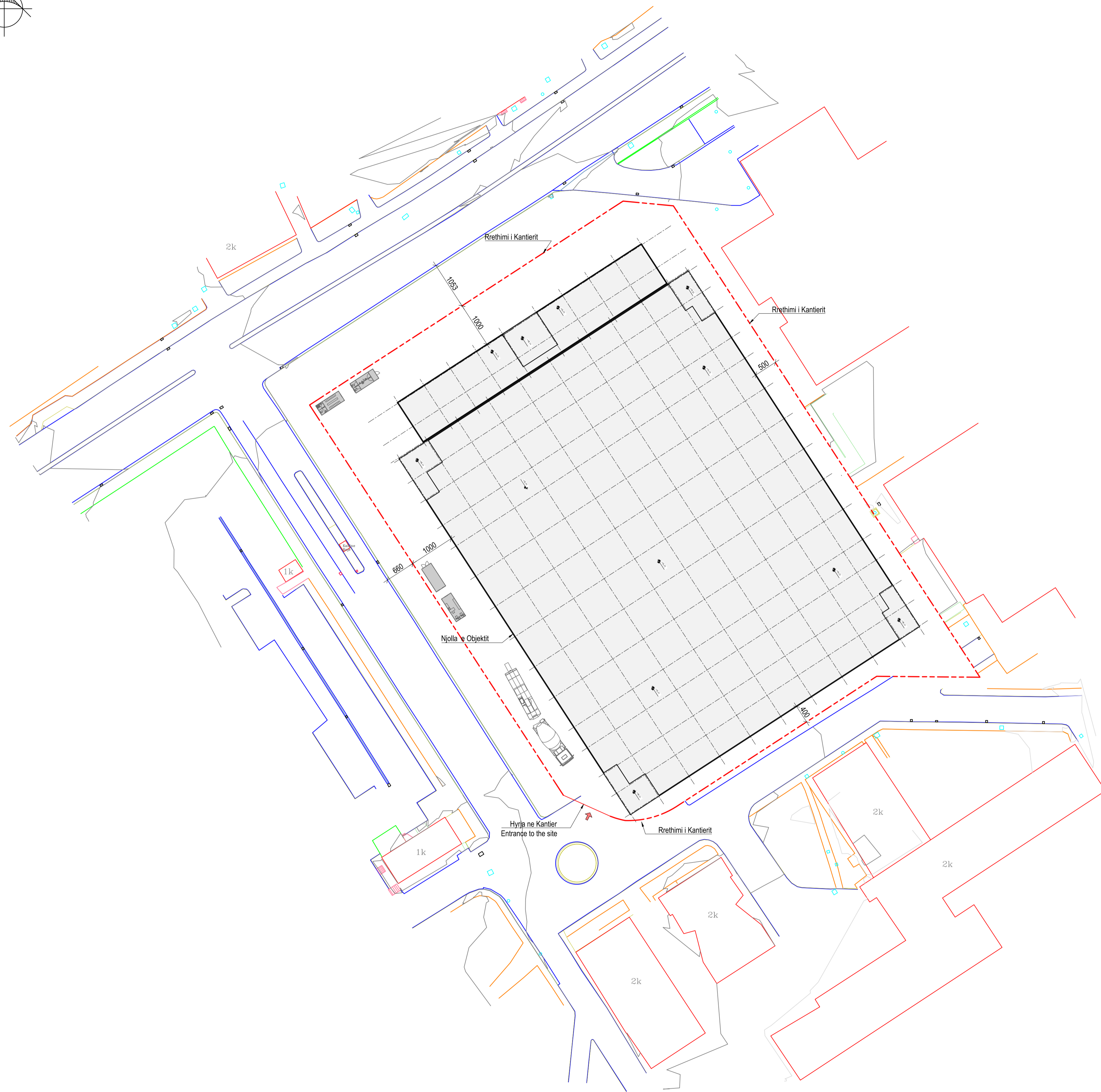
Plani i Organizimit të Kantierit Site Organization Plan 1 : 500
