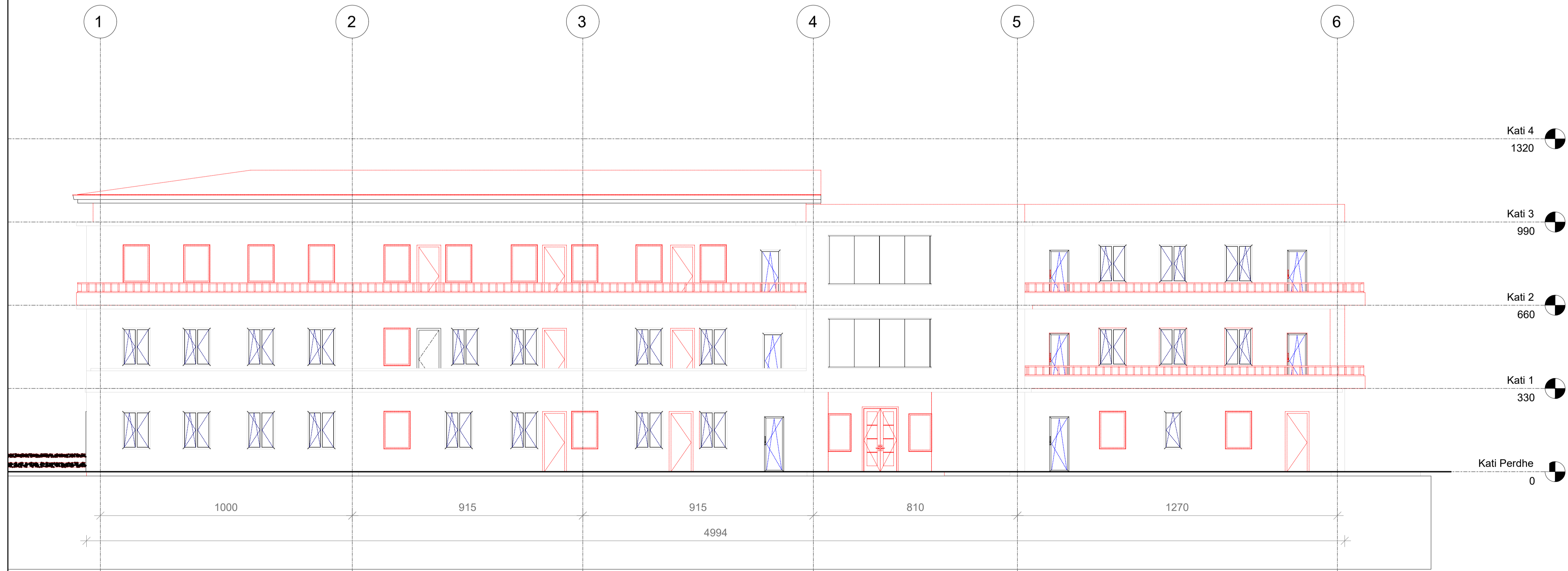
FASADA JUGORE
