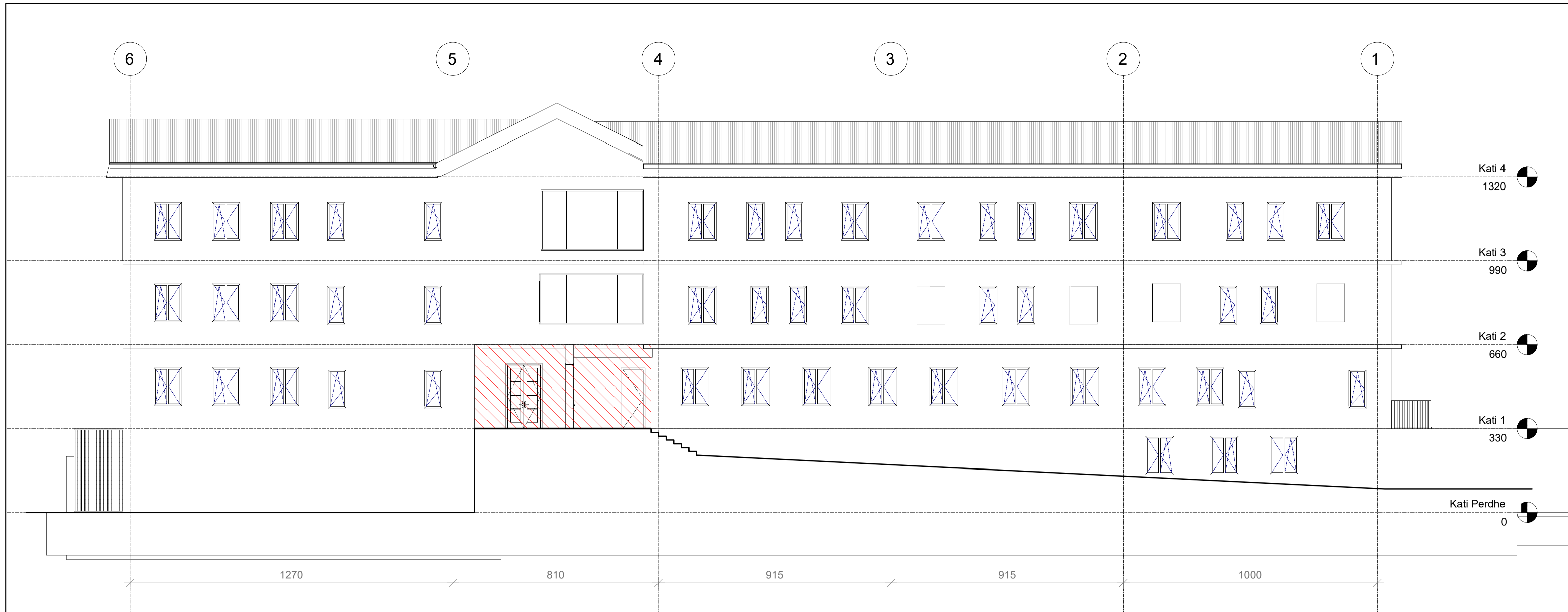
FASADA VERIORE
