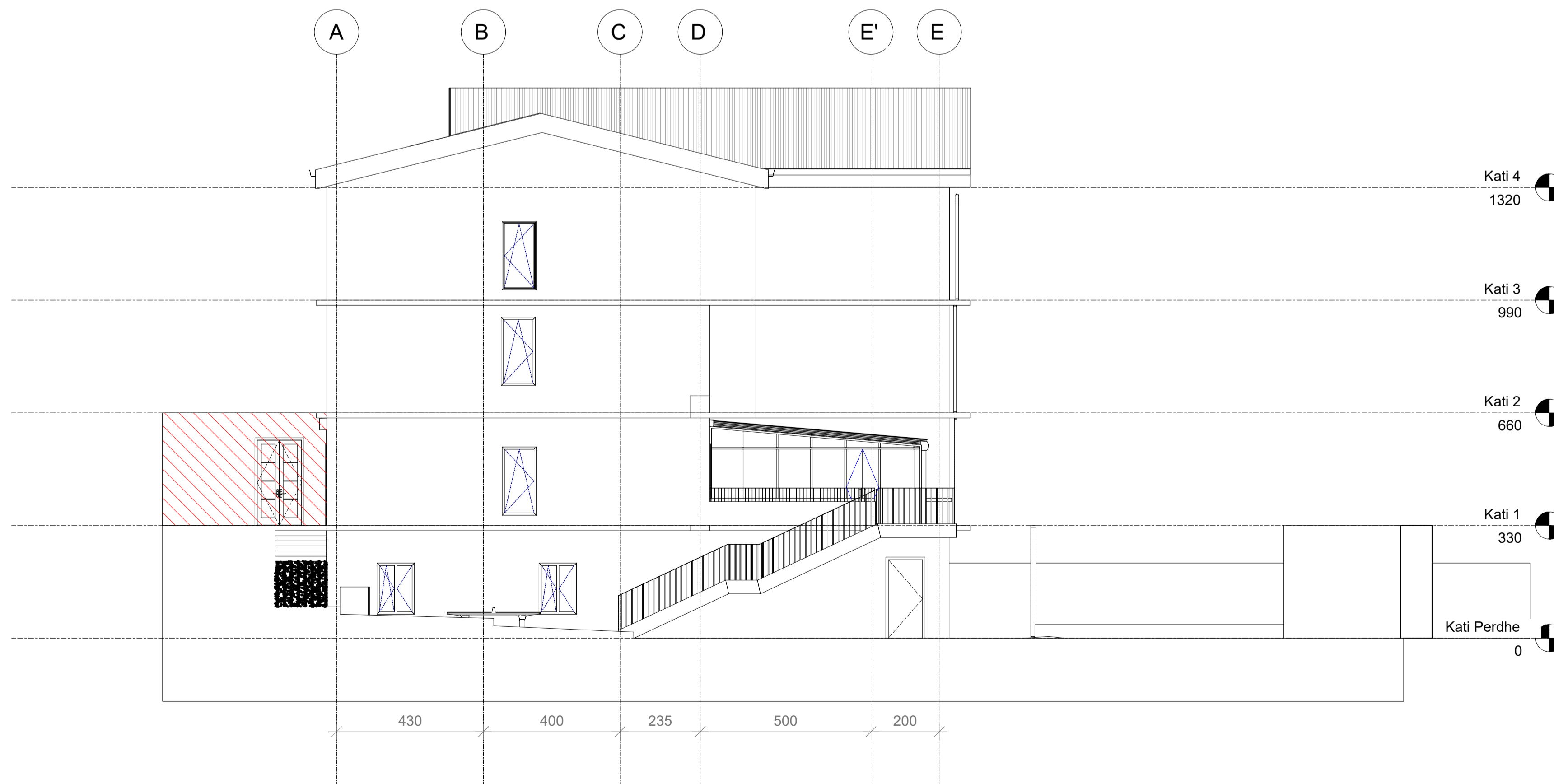
FASADA PERENDIMORE
