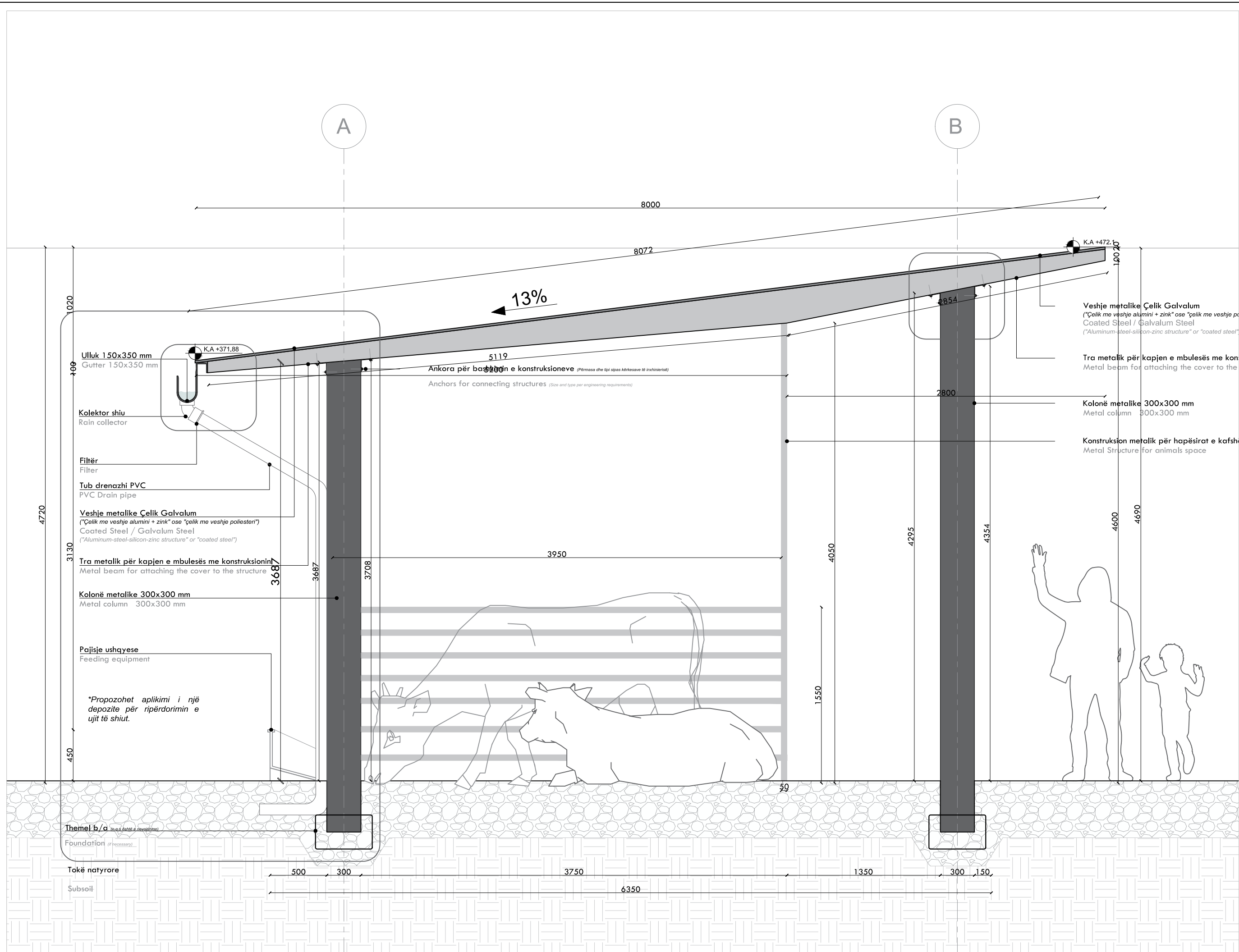
PRERJE A-A_MENYRA TRADICIONALE E DRENAZHIMIT
