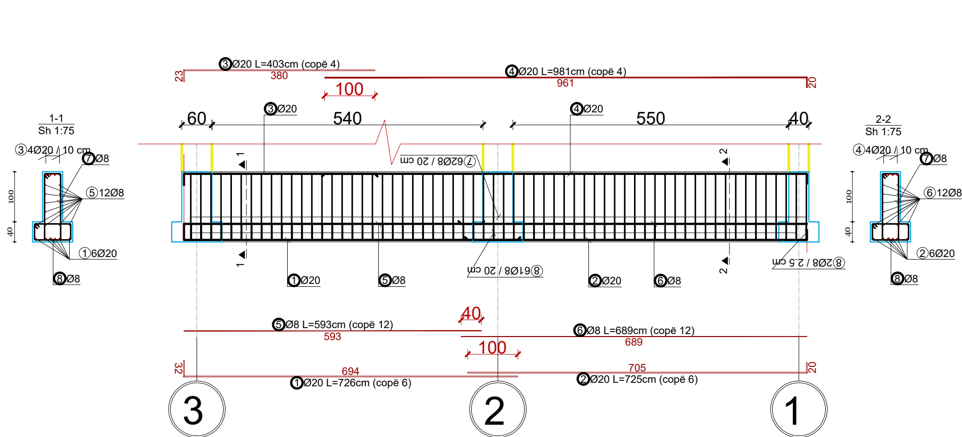
AKSI A-A, Tra themeli T-2
