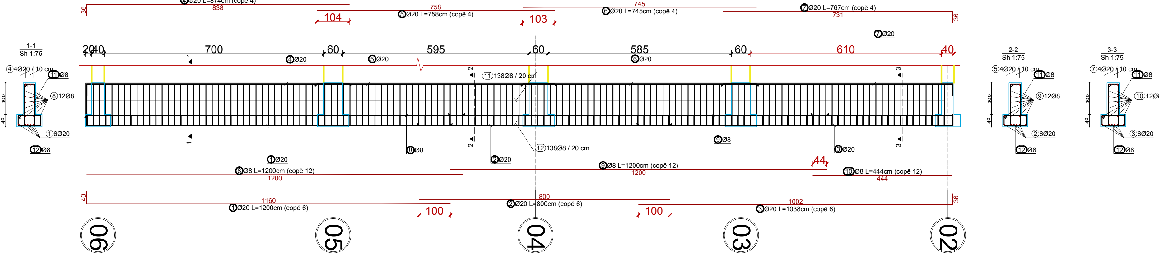
AKSI D-D, Tra themeli T-2
