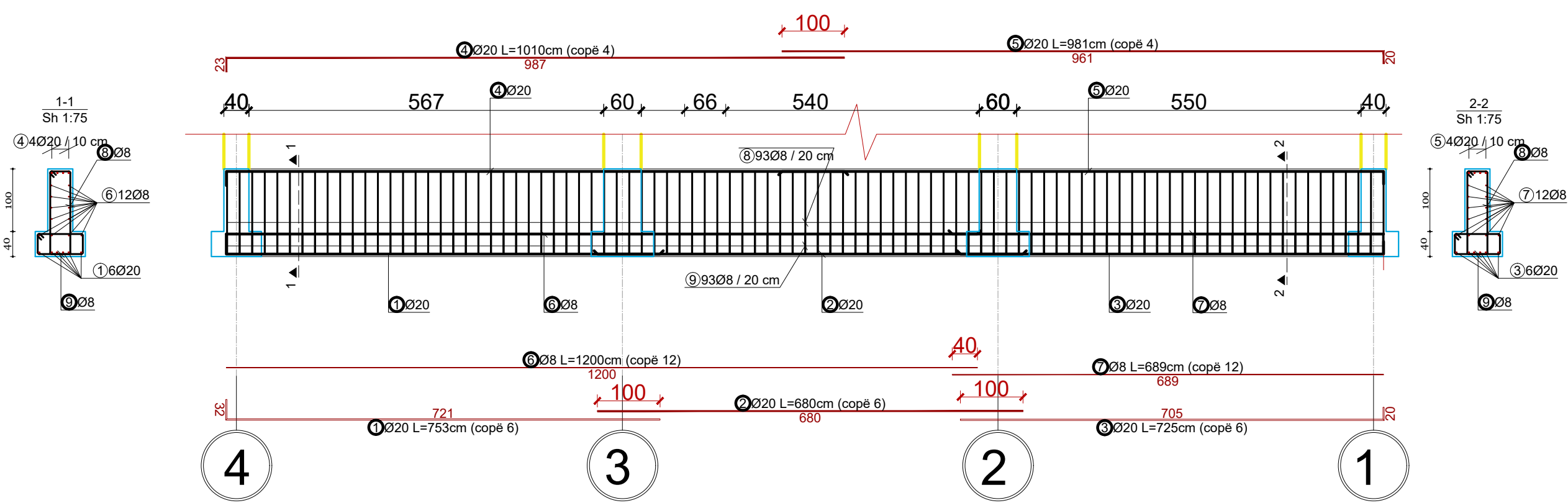
AKSI B-B, Tra themeli T-2
