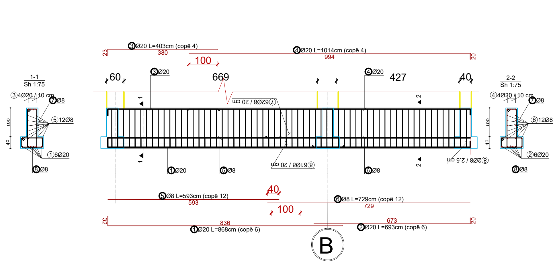
AKSI B-A-1, Tra themeli T-2
