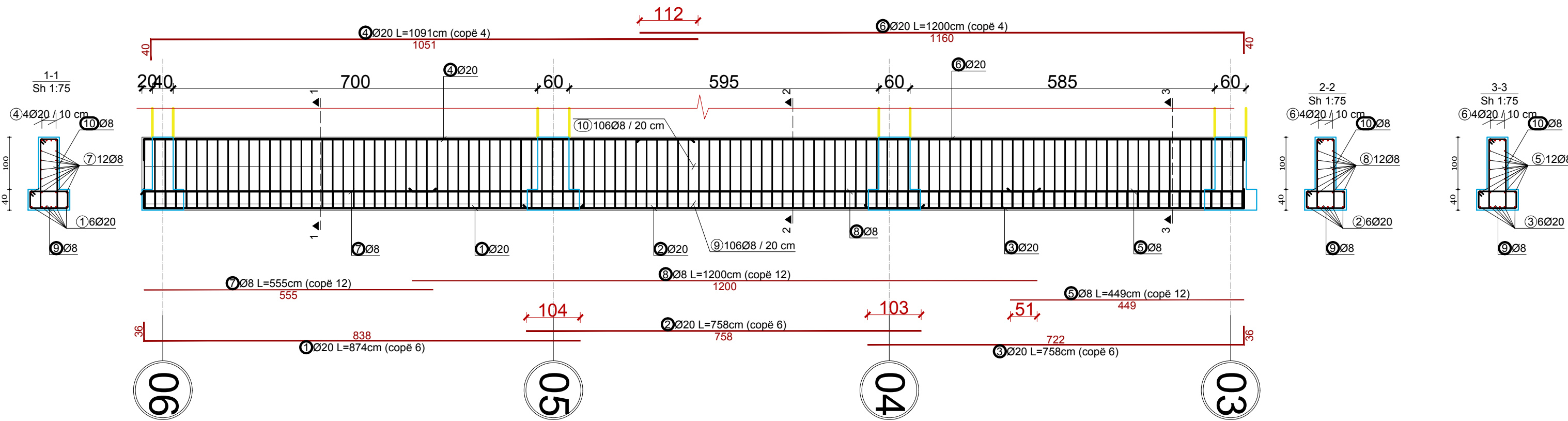
AKSI B-B, Tra themeli T-2
