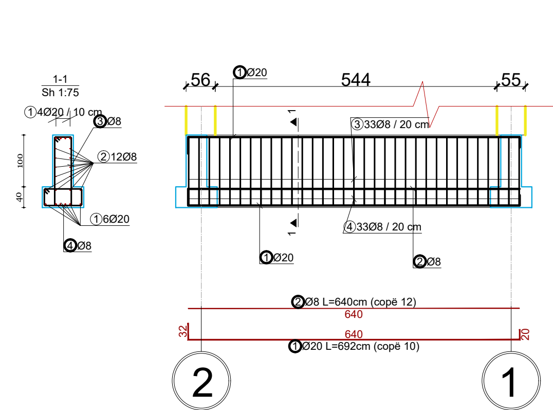
AKSI D-2-1, Tra themeli T-2
