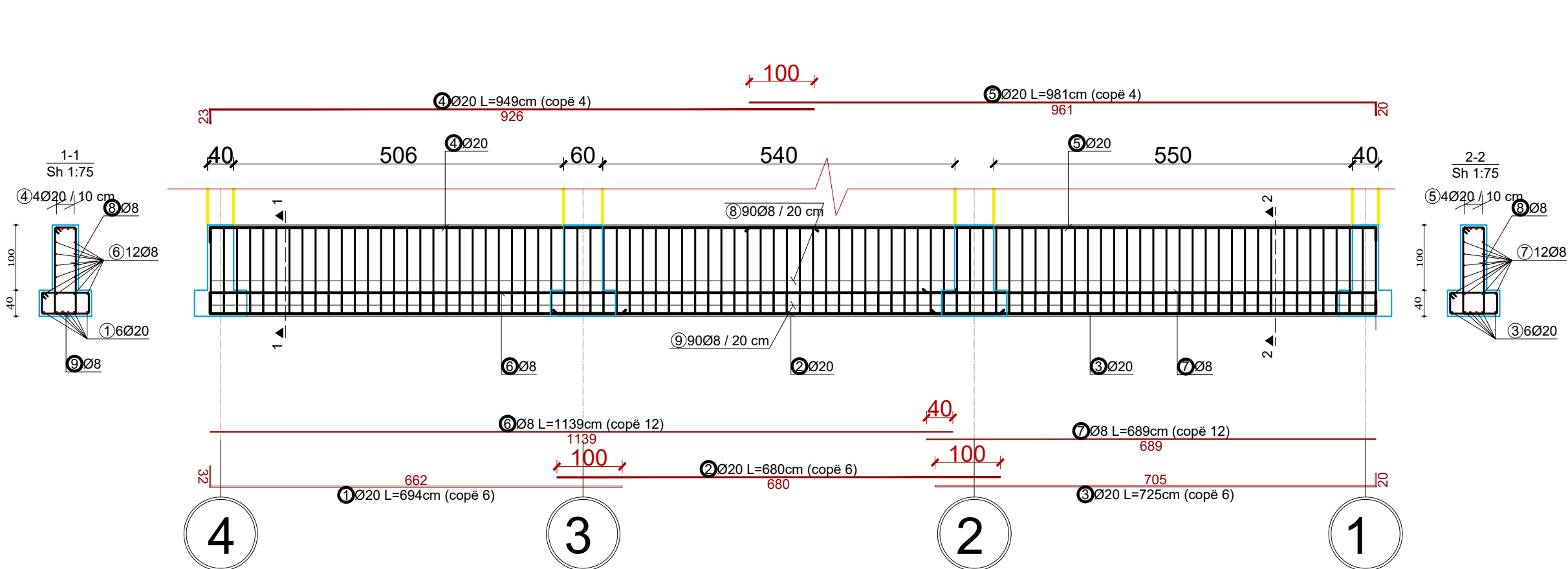
AKSI C-C, Tra themeli T-2
