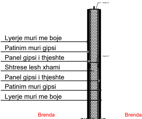
Detaj - Mur gipsi ambiente brend.
