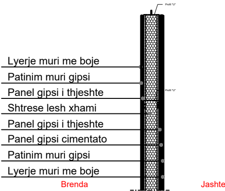
Detaj - Mur gipsi per ambiente jasht
