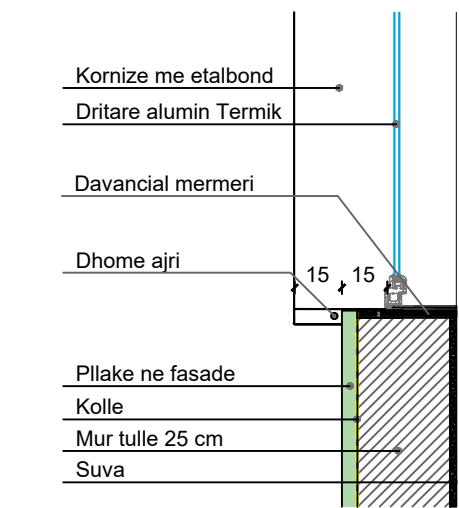
Detaji - Veshjes se kornizes se dritareve
