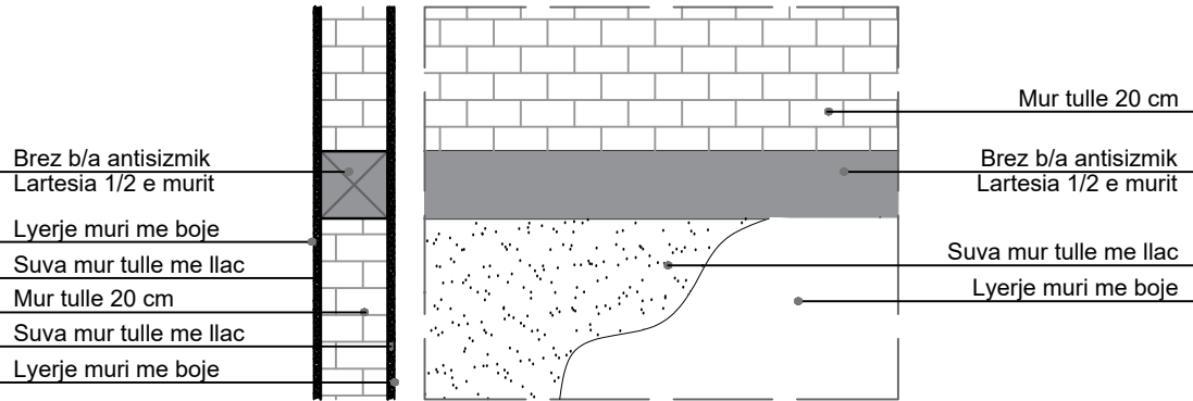
Detaj - Mur tulle dhoma teknike
