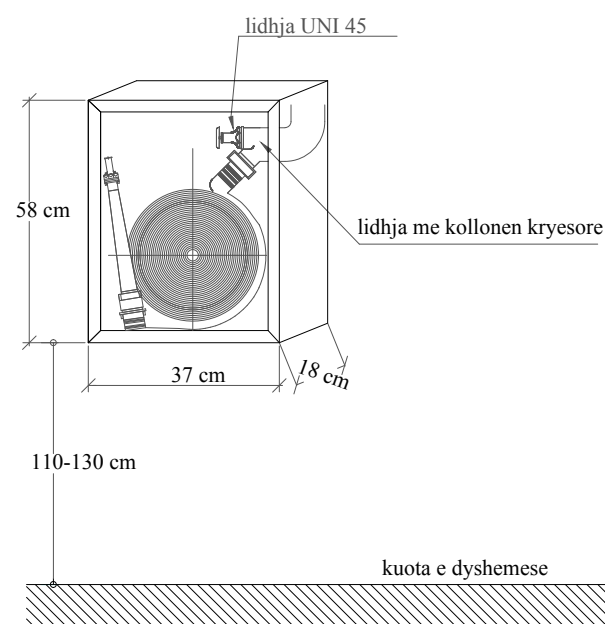
Hidranti me kasete ne mur
