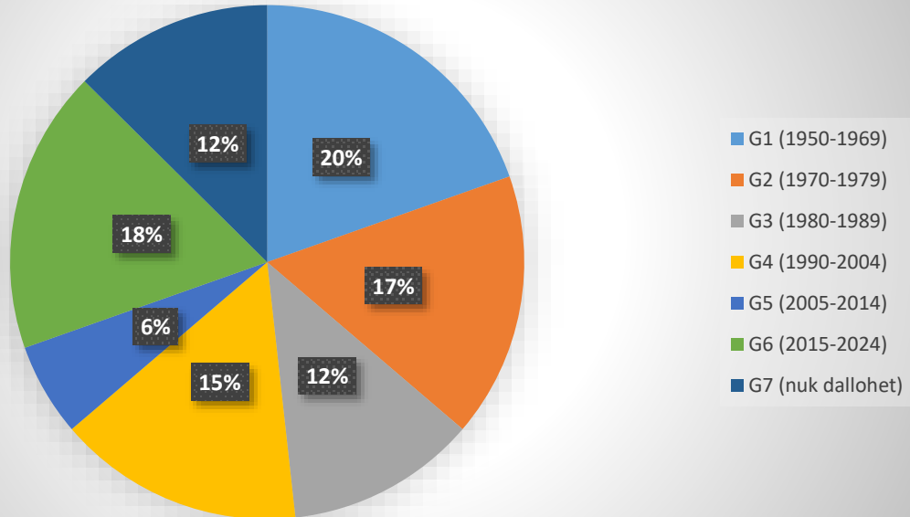
Paraqitje grafike viteve në punë të transformatorëve të fuqisë
