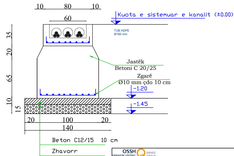
PRERJA B - B
