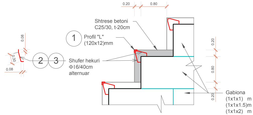
Shkallet e kaperderdhesit me pllaka betoni (1x2)m - konstrukcion hekuri / ml
