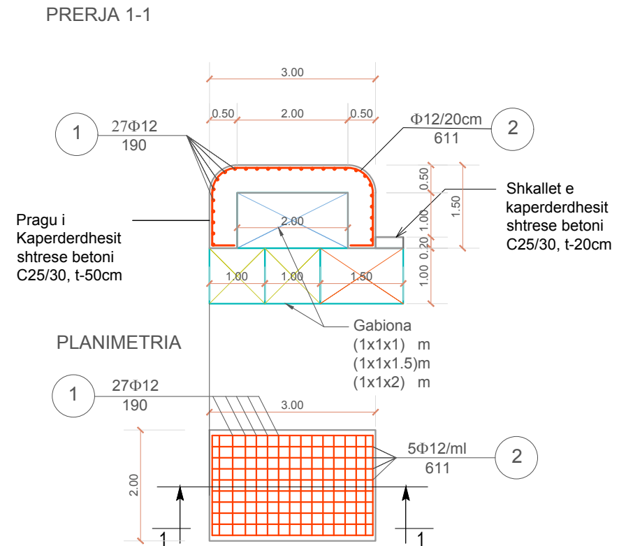
Pragu i Kaperderdhesit (3x2x0,5)m - armatura e hekurit / cope
