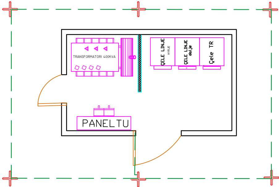
PLANIMETRIA E RIKONSTRUKSIONIT TE KABINES "THANAS ZIKO 1" FIDERI A3 NENSTACIONI RAJONAL TR 400KVA 20\0.4 KV
