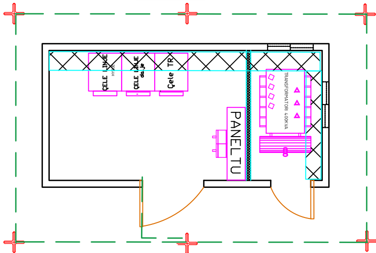
PLANIMETRIA E RIKONSTRUKSIONIT TE KABINES "K12/3" FIDERI A22 NENSTACIONI RAJONAL TR 400KVA 20\0.4 KV
