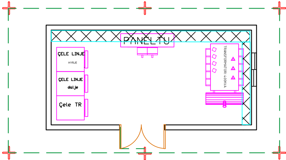
PLANIMETRIA E RIKONSTRUKSIONIT TE KABINES "S.ZORBA 1/FC.4" TR 630 KVA 20\0.4 KV
