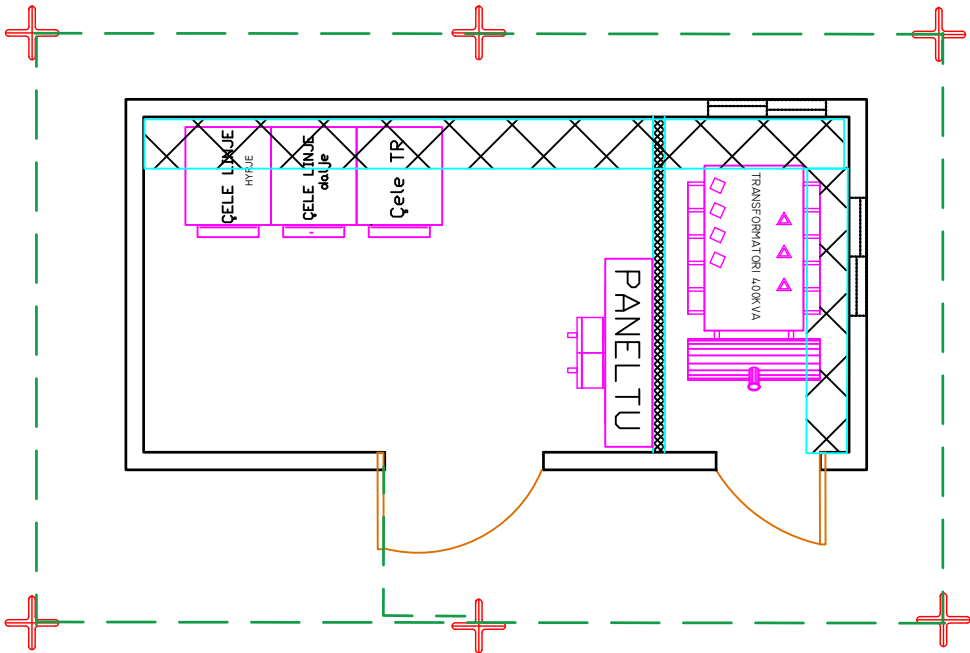
PLANIMETRIA E RIKONSTRUKSIONIT TE KABINES "K7" FIDERI A22 NENSTACIONI RAJONAL TR 400KVA 20\0.4 KV
