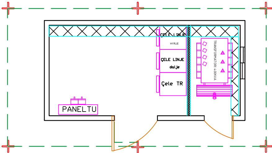
PLANIMETRIA E RIKONSTRUKSIONIT TE KABINES "K12/2 A22" TR 250 KVA 20\0.4 KV
