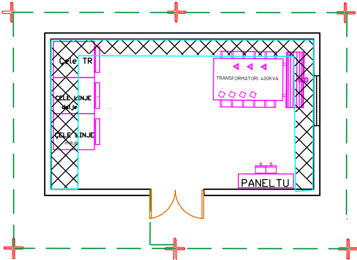
PLANIMETRIA E RIKONSTRUKSIONIT TE KABINES "K3" FIDERI A15 RAJONAL TR 400 KVA 20\0.4 KV
