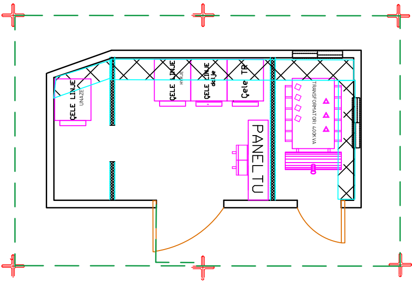
PLANIMETRIA E RIKONSTRUKSIONIT TE KABINES "K3" FIDERI A21 NENSTACIONI RAJONAL TR 400KVA 20\0.4 KV
