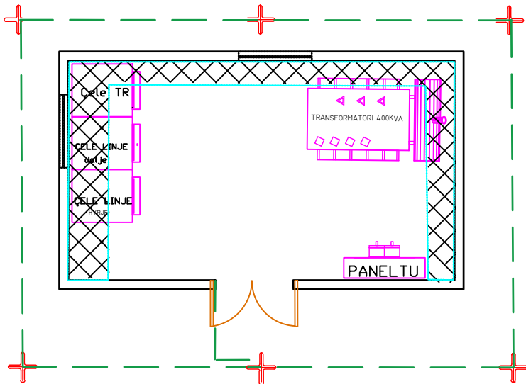
PLANIMETRIA E RIKONSTRUKSIONIT TE KABINES "K4" FIDERI A15 RAJONAL TR 400 KVA 20\0.4 KV
