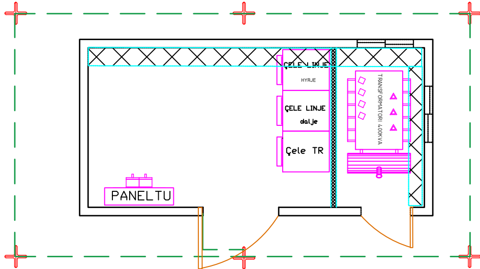
PLANIMETRIA E RIKONSTRUKSIONIT TE KABINES "K2/A21" TR 250 KVA 20\0.4 KV
