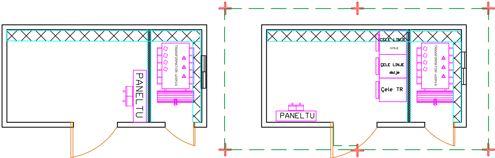
PLANIMETRIA E RIKONSTRUKSIONIT TE KABINES "K19/F355" TR 400 KVA 20\0.4 KV
