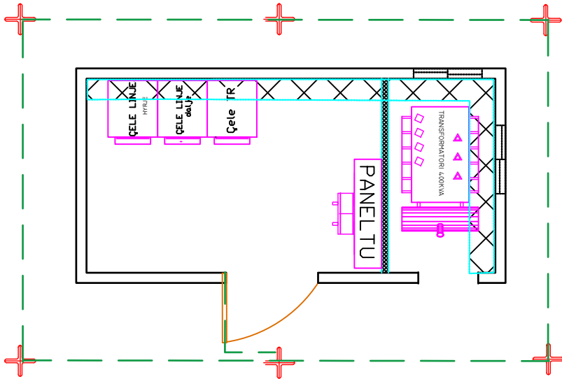
PLANIMETRIA E RIKONSTRUKSIONIT TE KABINES "K5" FIDERI A23 NENSTACIONI RAJONAL TR 400KVA 20\0.4 KV
