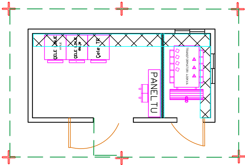
PLANIMETRIA E RIKONSTRUKSIONIT TE KABINES "K1" FIDERI A22 NENSTACIONI RAJONAL TR 400KVA 20\0.4 KV
