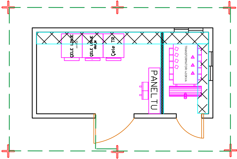
PLANIMETRIA E RIKONSTRUKSIONIT TE KABINES "K10" FIDERI A21 NENSTACIONI RAJONAL TR 400KVA 20\0.4 KV
