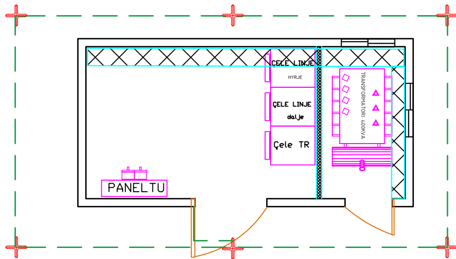
PLANIMETRIA E RIKONSTRUKSIONIT TE KABINES "K3/A22" TR 250 KVA 20\0.4 KV
