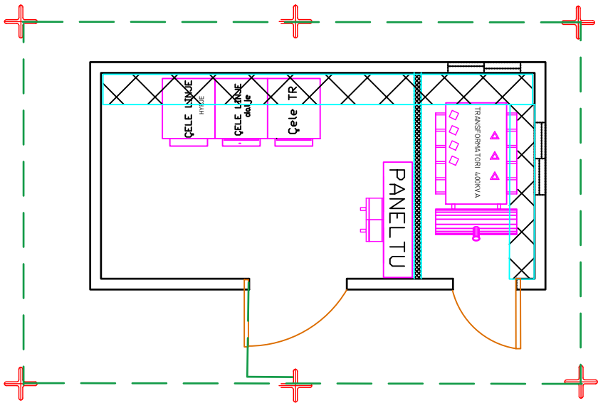
PLANIMETRIA E RIKONSTRUKSIONIT TE KABINES "K5" FIDERI A22 NENSTACIONI RAJONAL TR 400KVA 20\0.4 KV
