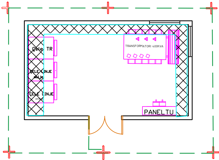
PLANIMETRIA E RIKONSTRUKSIONIT TE KABINES "K9/1" FIDERI A15 RAJONAL TR 400 KVA 20\0.4 KV
