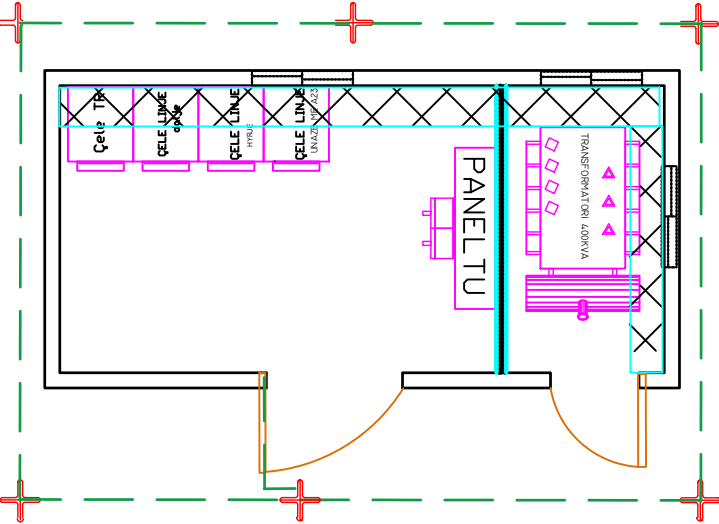
PLANIMETRIA E RIKONSTRUKSIONIT TE KABINES "K10" FIDERI A22 RAJONAL TR 400 KVA 20\0.4 KV
