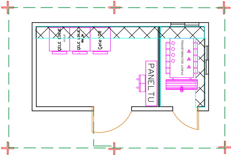
PLANIMETRIA E RIKONSTRUKSIONIT TE KABINES "K4" FIDERI A23 NENSTACIONI RAJONAL TR 400KVA 20\0.4 KV
