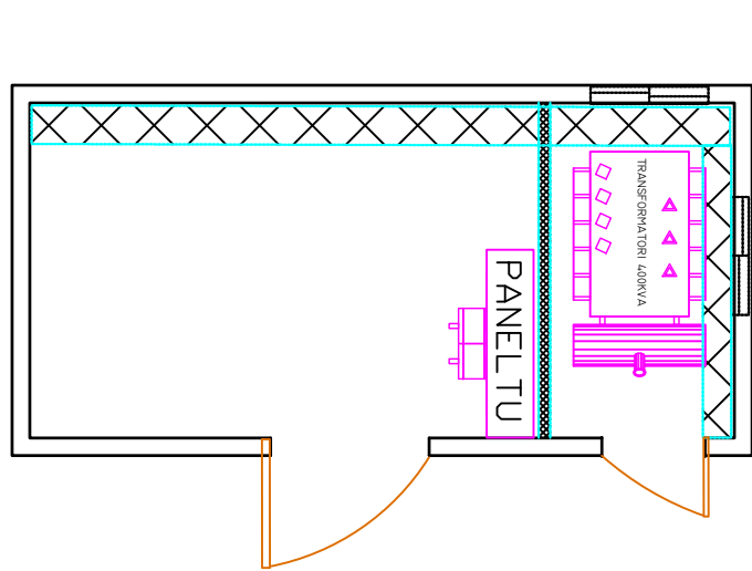
PLANIMETRIA EKZISTUESE KABINES "K3/A22" TR 250 KVA 20\0.4 KV
