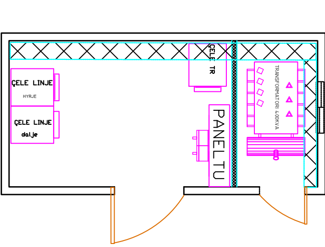
PLANIMETRIA EKZISTUESE KABINES "K12/2 A22" TR 250KVA 20\0.4 KV
