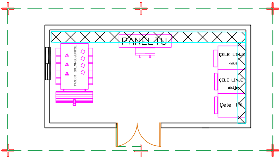
PLANIMETRIA E RIKONSTRUKSIONIT TE KABINES "MAGAZINA E TREGTISE FA1" TR 800KVA 20\0.4 KV
