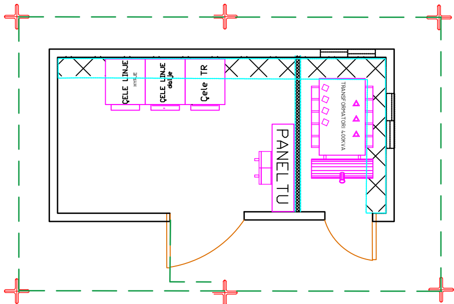
PLANIMETRIA E RIKONSTRUKSIONIT TE KABINES "K15" FIDERI A22 NENSTACIONI RAJONAL TR 400KVA 20\0.4 KV
