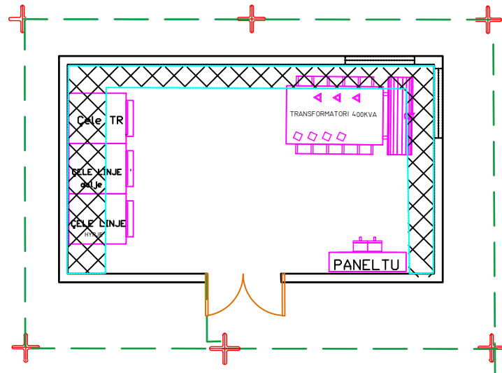
PLANIMETRIA E RIKONSTRUKSIONIT TE KABINES "K11" FIDERI A15 RAJONAL TR 400 KVA 20\0.4 KV
