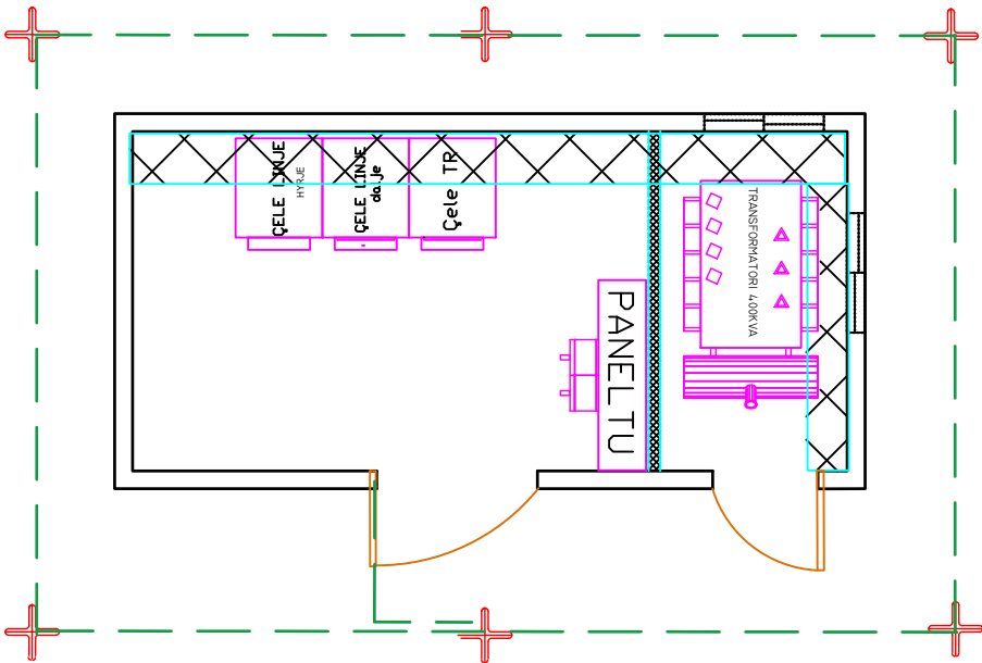
PLANIMETRIA E RIKONSTRUKSIONIT TE KABINES "K12/1" FIDERI A22 NENSTACIONI RAJONAL TR 400KVA 20\0.4 KV
