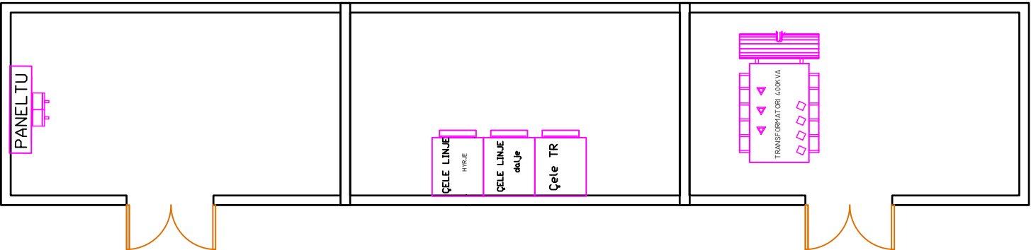
PLANIMETRIA E RIKONSTRUKSIONIT TE KABINES "KONVIKTI 1" TR 400KVA 20\0.4 KV
