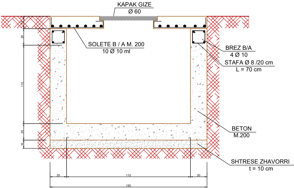
PRERJA TERTHORE SH1:25
