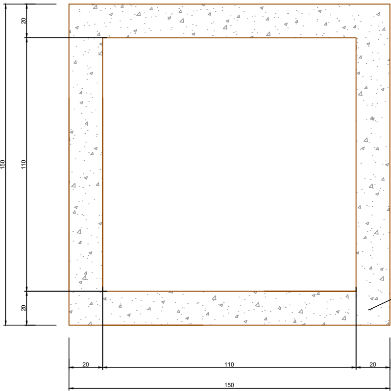
PLANIMETRIA SH1:25
