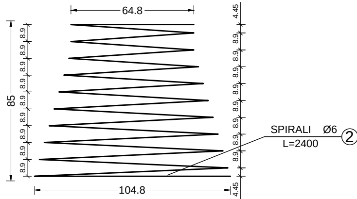
SPIRALI BRENDESHEM
