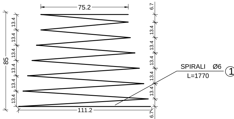
SPIRALI BRENDESHEM
