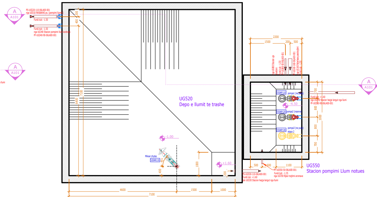
4 plan -1.00 1 : 50
