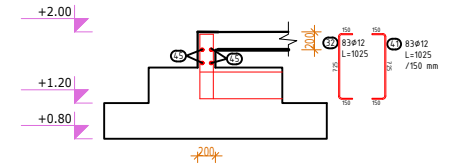
Armimi i Murit Aksi 1-1, 3-3 Sh 1:30
