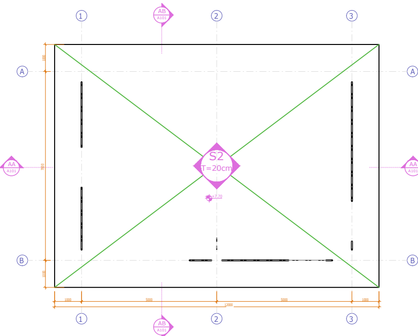
Armimi i Soletes S2 Kuota +7.70 SH.1:50
