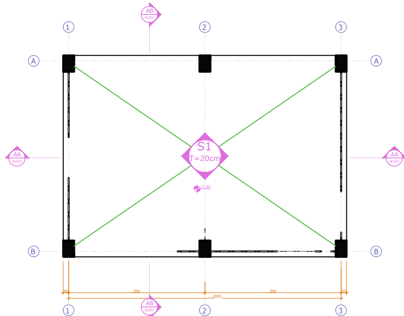
Armimi i Soletes S1 Kuota +1.80 SH.1:50
