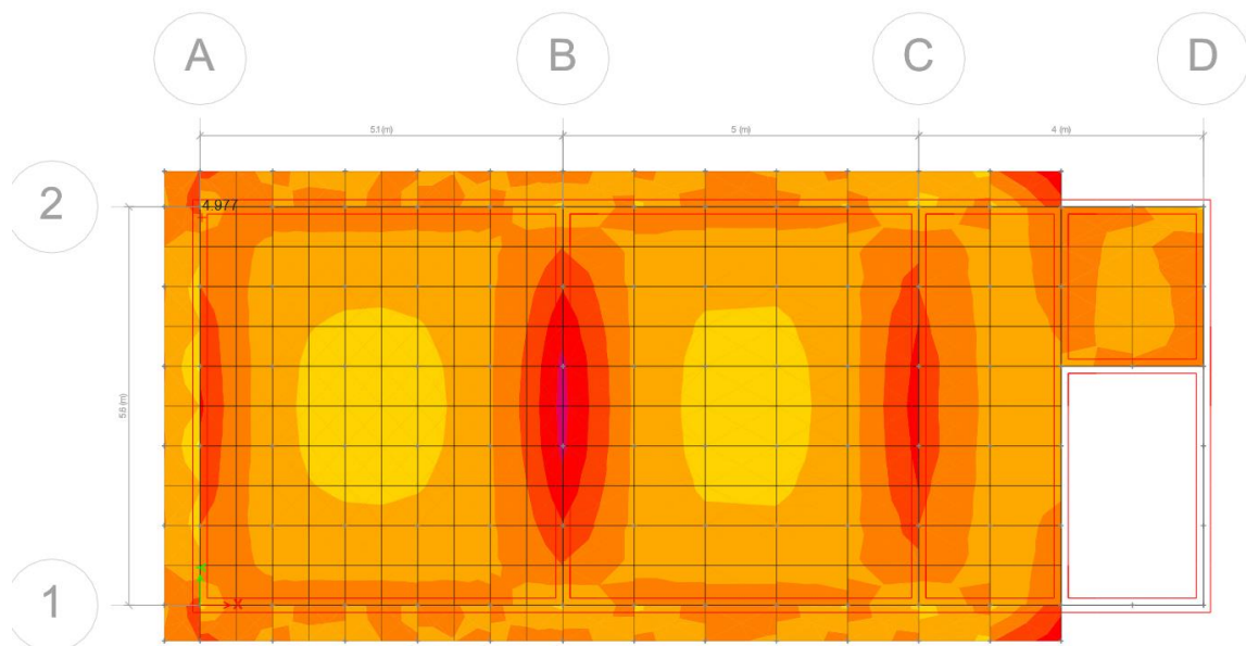
Figura 7 – Momenti perkules sipas X ne kNm per kombinimet ULS, M_{max}=64 \text{ kNm/m}
