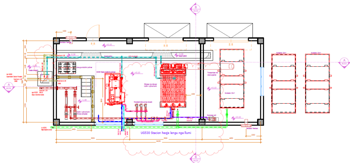
Figura 1 – Planimetria e godines
