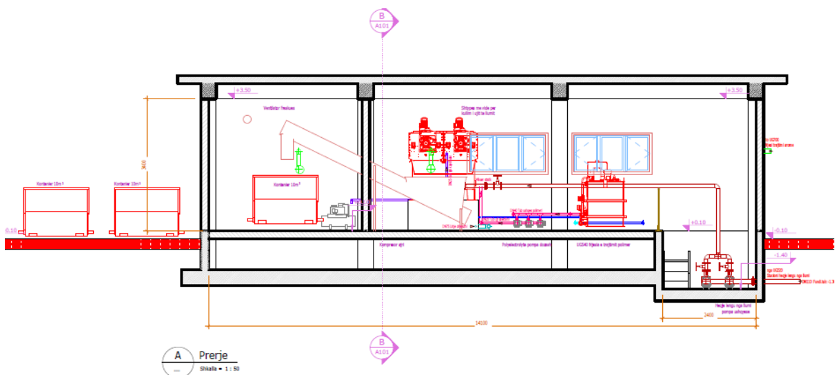
Figura 2 – Prerja gjatesore e godines
