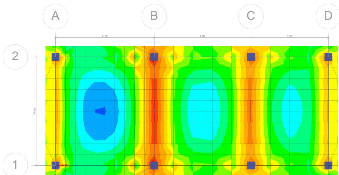
Figura 12 – Momenti perkules sipas X ne kNm/m per kombinimin ULS, M_{max}=21 kNm/m
