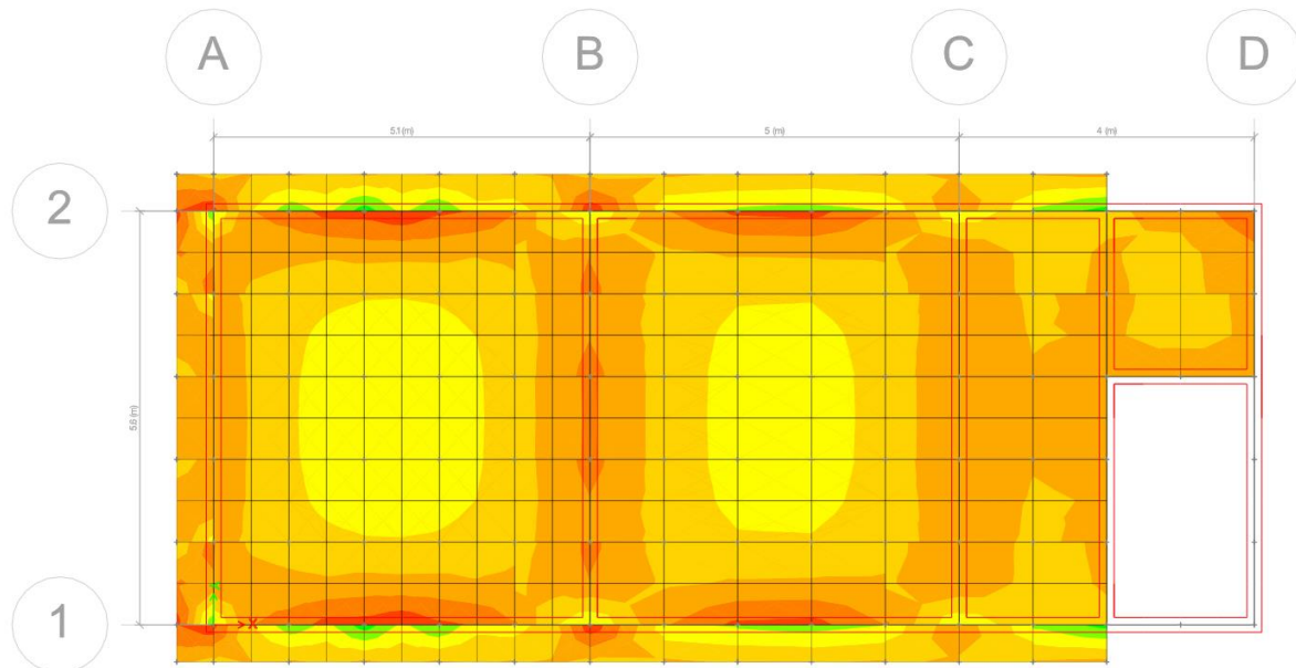
Figura 6 – Momenti perkules sipas Y ne kNm per kombinimet ULS, M_{max}=40 kNm/m
