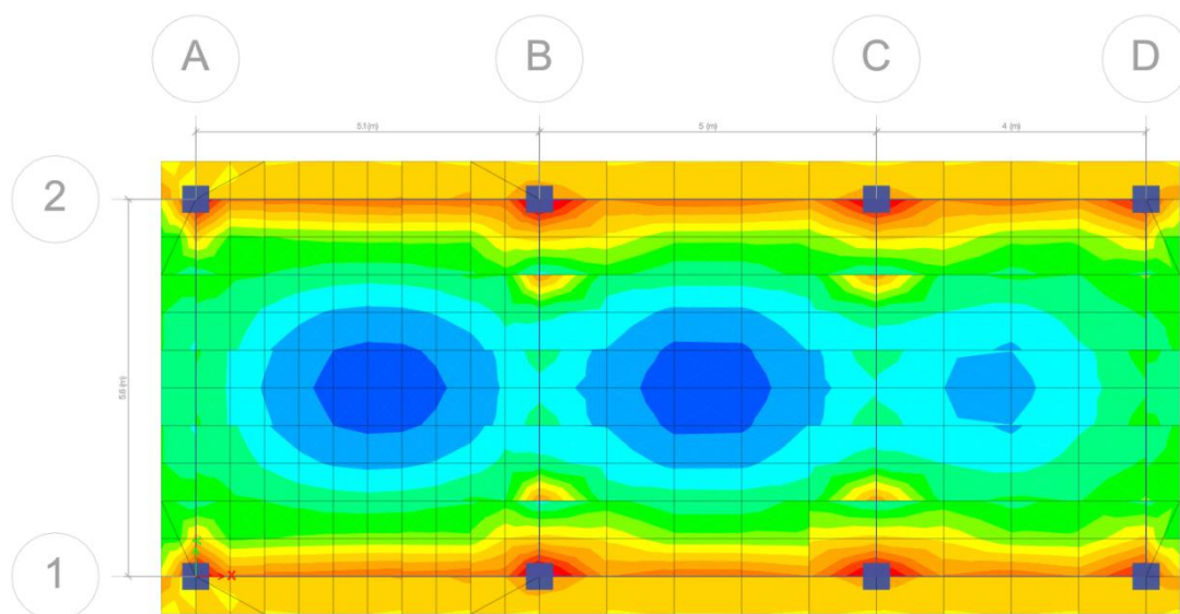
Figura 11 – Momenti perkules sipas Y ne kNm/m per kombinimin ULS, M_{max}=21 kNm/m
