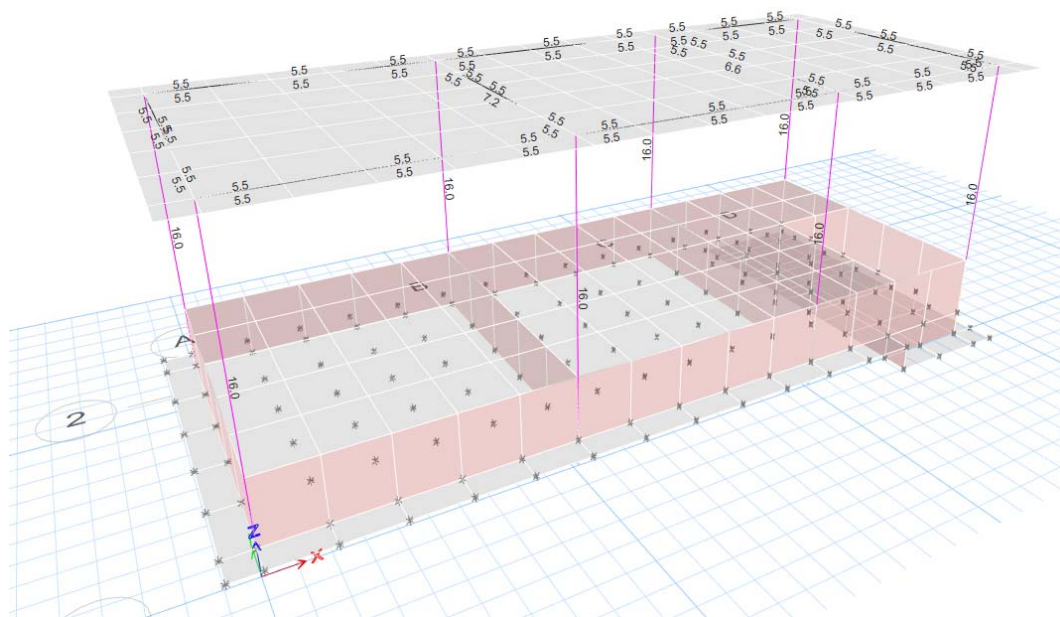
Figura 7 – Armimi i kolonave i shprehur ne \text{cm}^2
