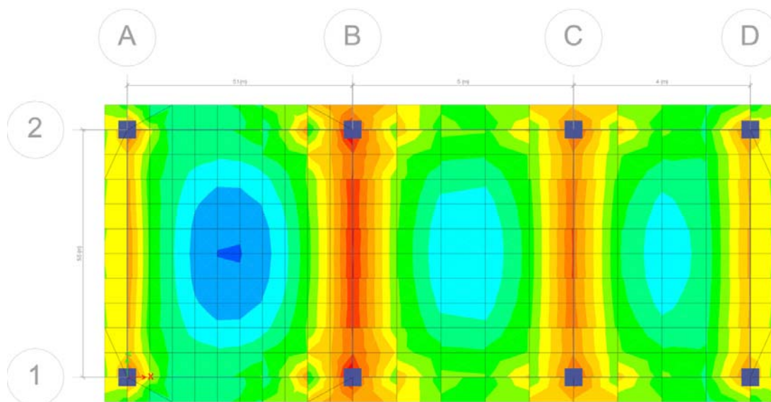
Figura 10 – Momenti perkules sipas X ne kNm/m per kombinimin ULS, M_{max}=18 kNm/m
