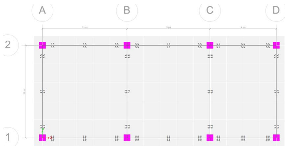
Figura 8 – Armimi i trareve i shprehur ne cm 2
