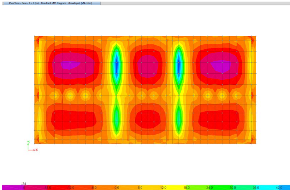
Figura 5 – Momenti perkules sipas X ne kNm per kombinimet ULS, M_{max}=54 \text{ kNm/m}
