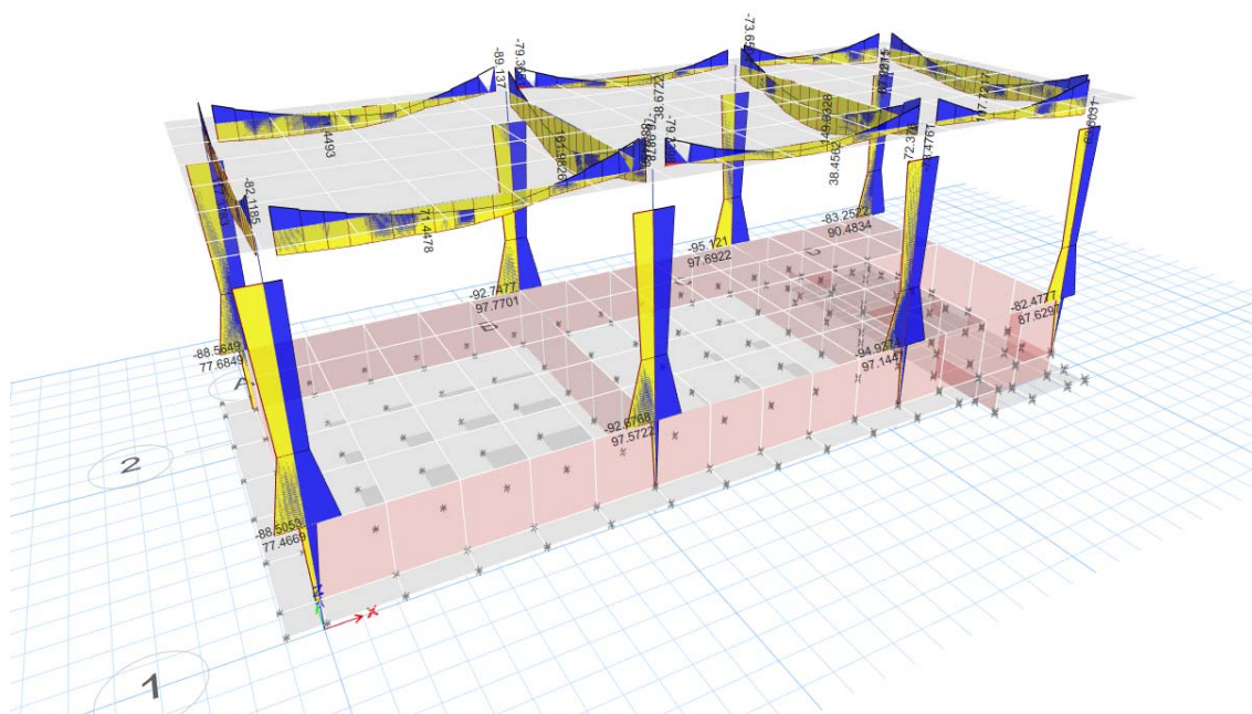
Figura 6 – Diagrama e momenteve perkules ne ne kolona ne kNm
