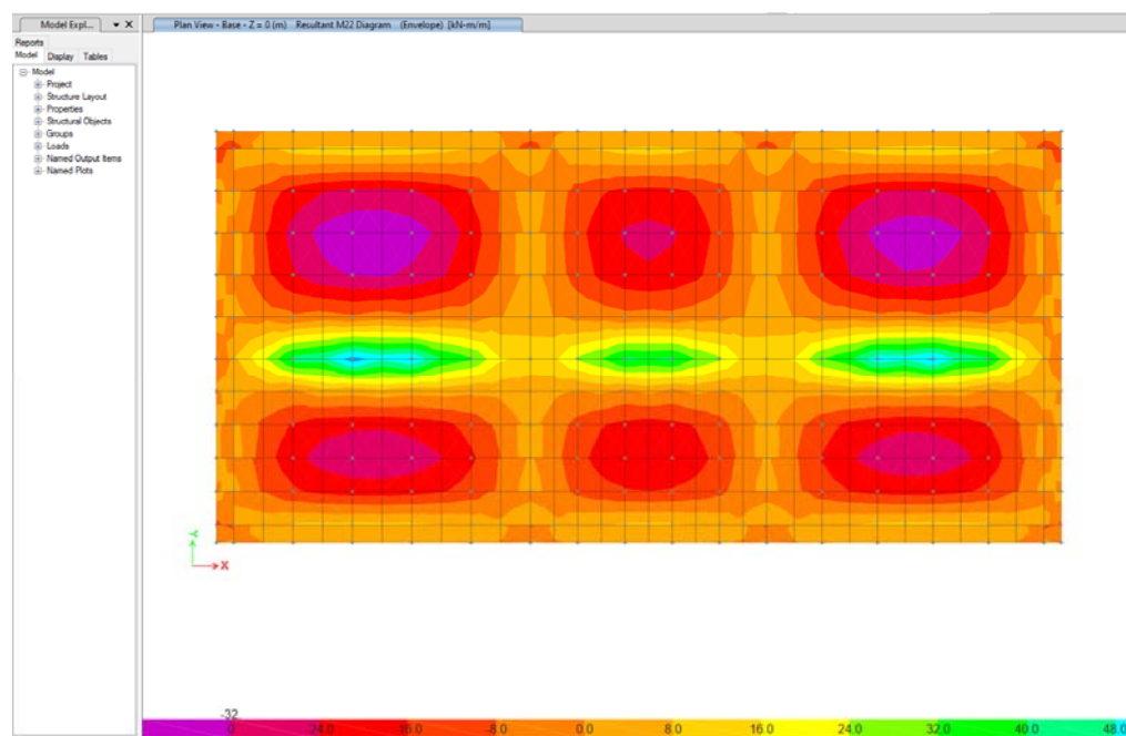
Figura 4 – Momenti perkules sipas Y ne kNm per kombinimet ULS, Mmax=40 kNm/m
