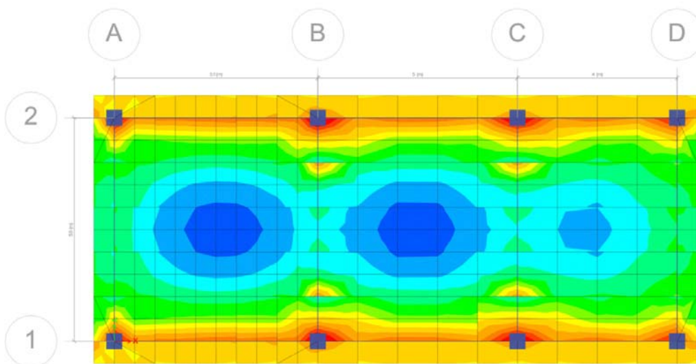
Figura 9 – Momenti perkules sipas Y ne kNm/m per kombinimin ULS, M_{max}=18 kNm/m
