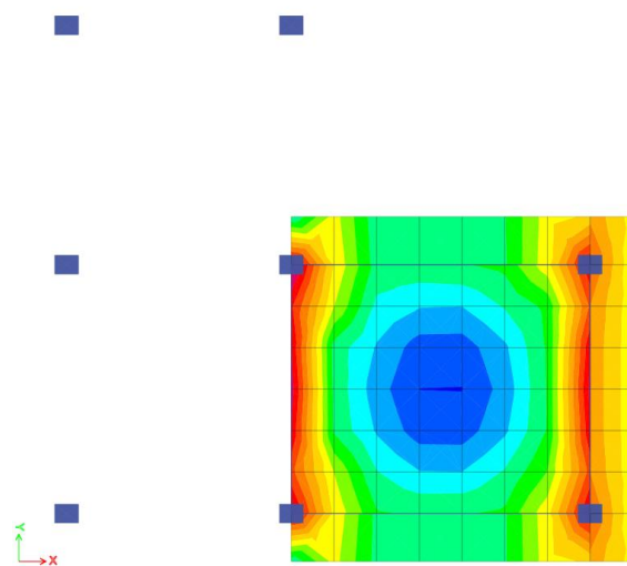
Figura 11 – Momenti perkules sipas X ne kNm/m per kombinimin ULS, M_{max}=15 kNm/m
