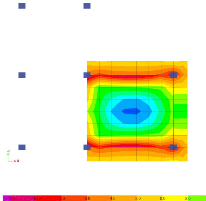
Figura 10 – Momenti perkules sipas Y ne kNm/m per kombinimin ULS, M_{max}=13 kNm/m
