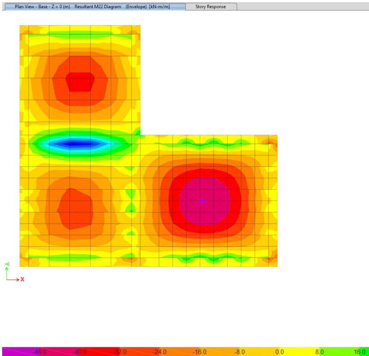
Figura 5 – Momenti perkules sipas Y ne kNm per kombinimet ULS, M_{max}=63 \text{ kNm/m}
