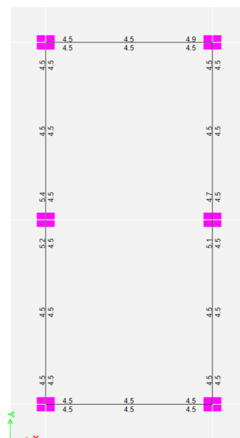
Figura 9 – Armimi i trareve i shprehur ne cm^2
