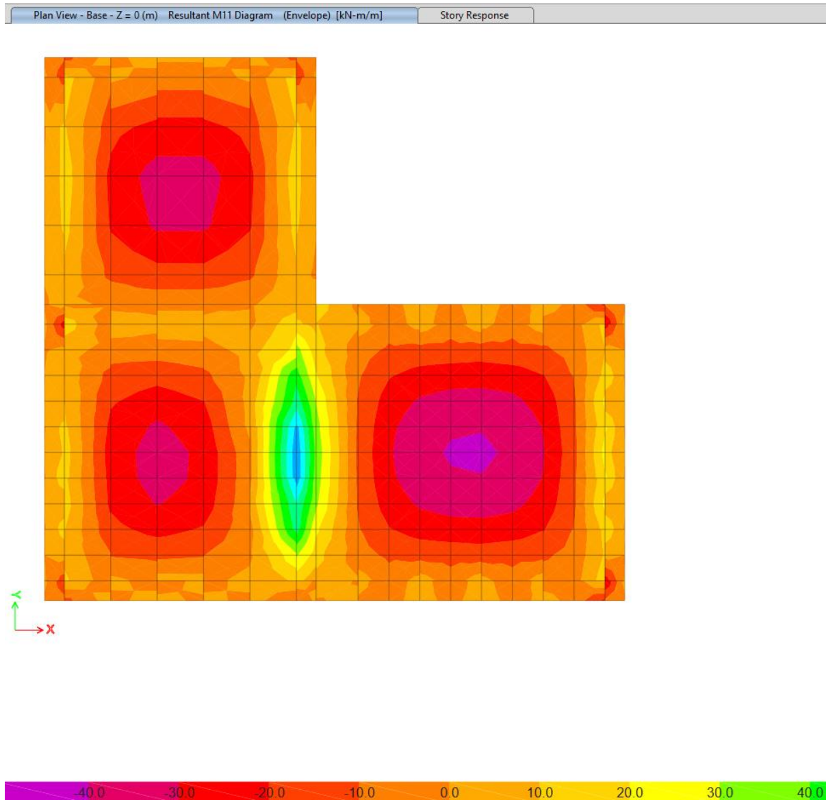
Figura 6 – Momenti perkules sipas X ne kNm per kombinimet ULS, M_{max}=78 kNm/m
