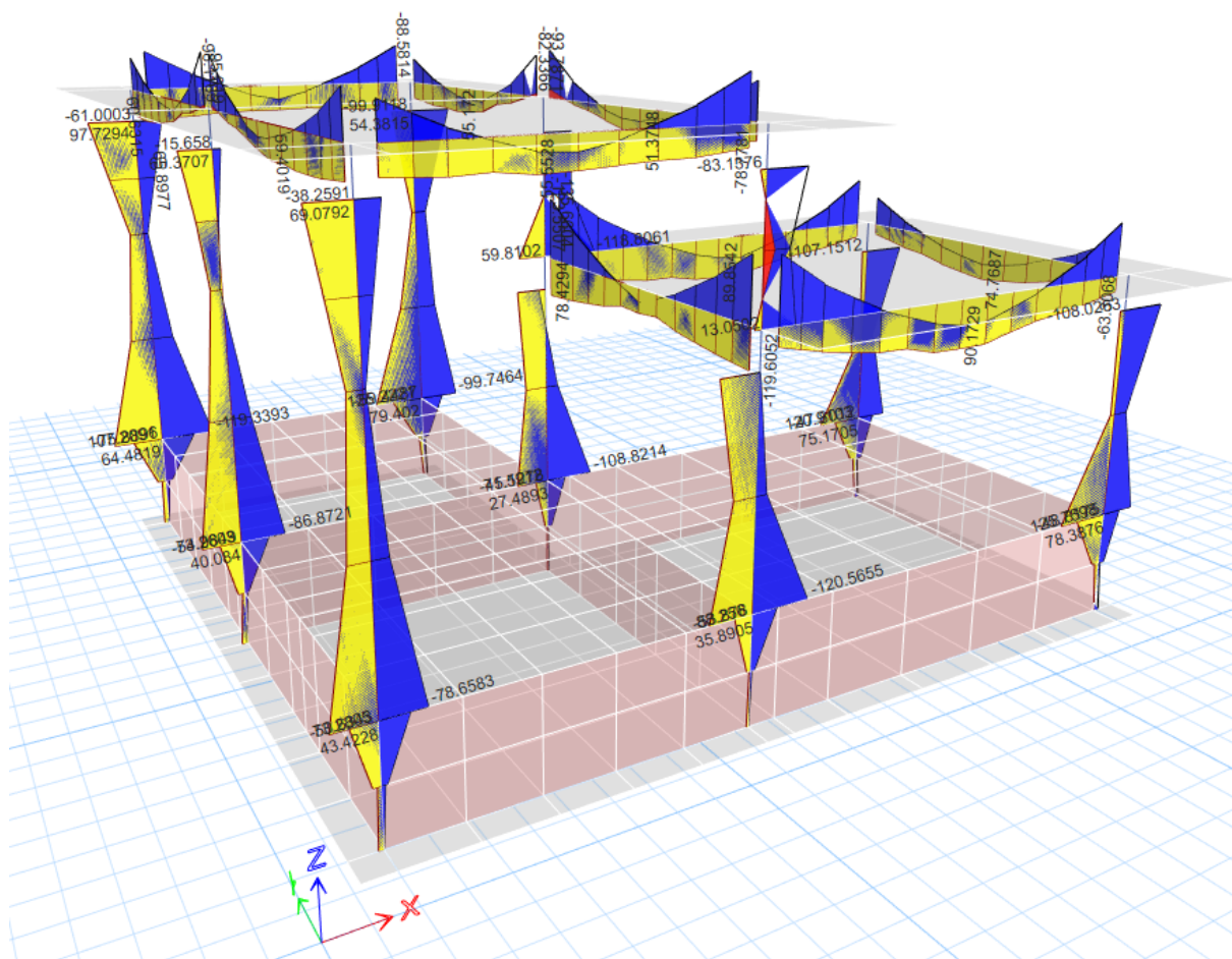
Figura 7 – Diagrama e momenteve perkules ne ne kolona ne kNm
