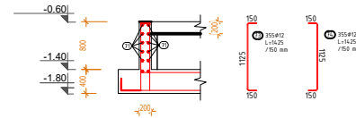
ARMIMI I MURIT SH 1:40
