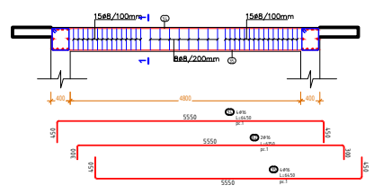
Armimi i Traut T8 (Cope 1) SH 1:50
