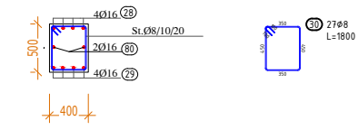
Prerja 1-1 trau T6 Sh 1:25
