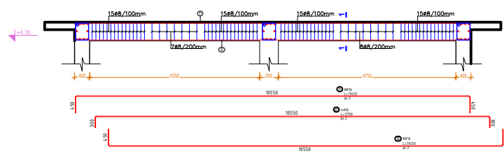
Armimi i Traut T8 (Cope 1) SH 1:50
