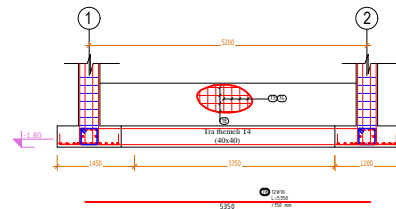
Armimi i Murit Aksi C-C SH. 1:50
