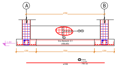
Armimi i Murit Aksi 3-3 SH. 1:50
