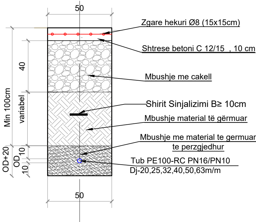
Shk 1:25
