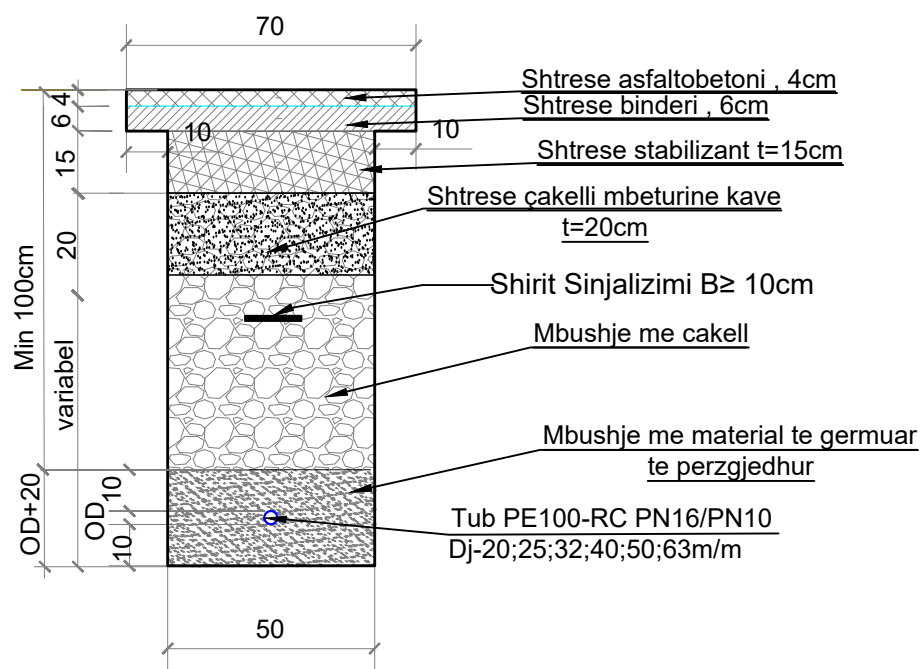
Shk 1:25
