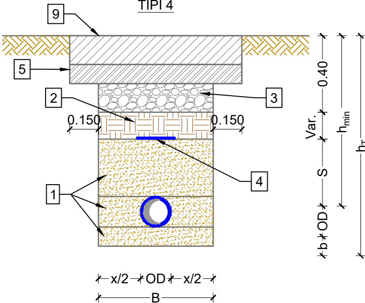
RRUGE BETONI TIPI 4
