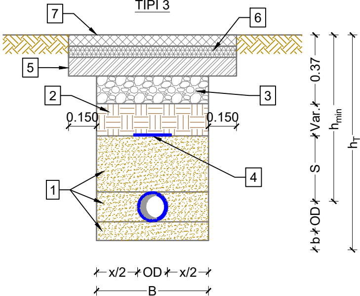
RRUGE ASFALTI TIPI 3
