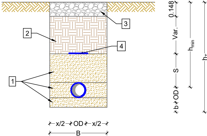
RRUGE TE PASHTRUARA TIPI 2
