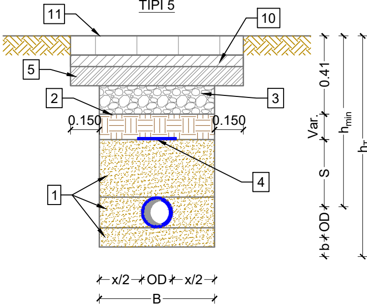
TROTUAR ME PLLAKA TIPI 5
