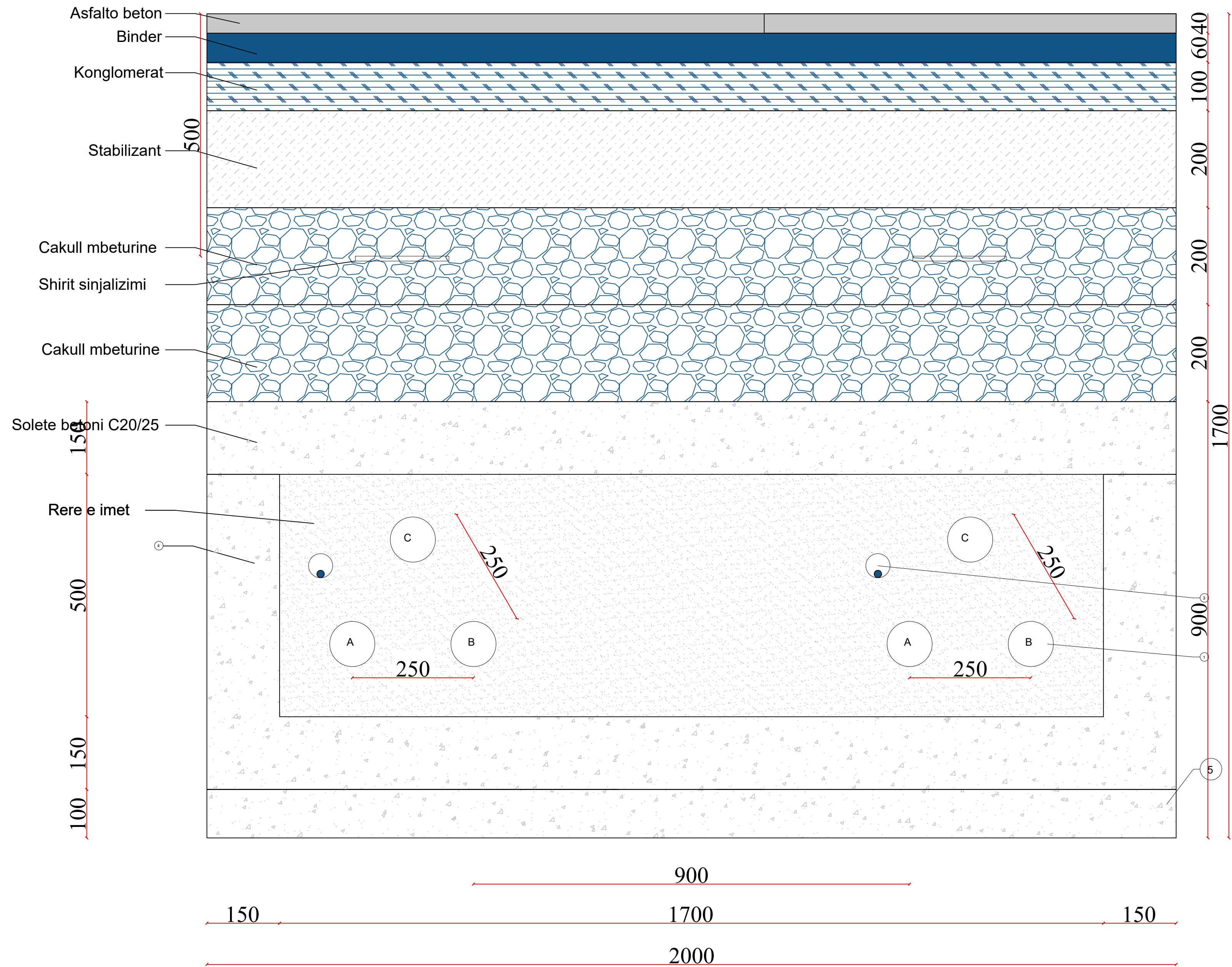
Tipi 2 me kanal betoni per dy qarqe linje (me asfalt)
