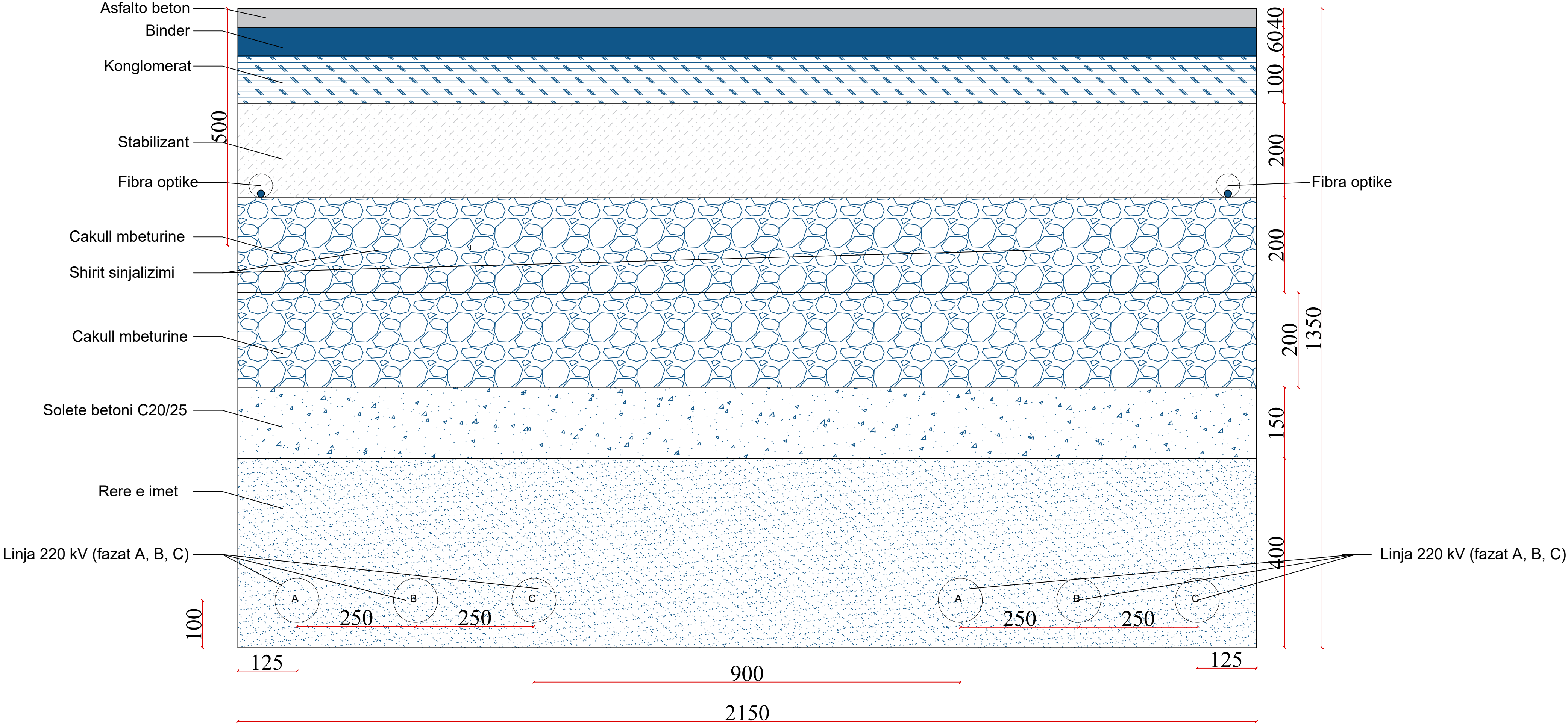
Tipi 1 (me asfalt)
