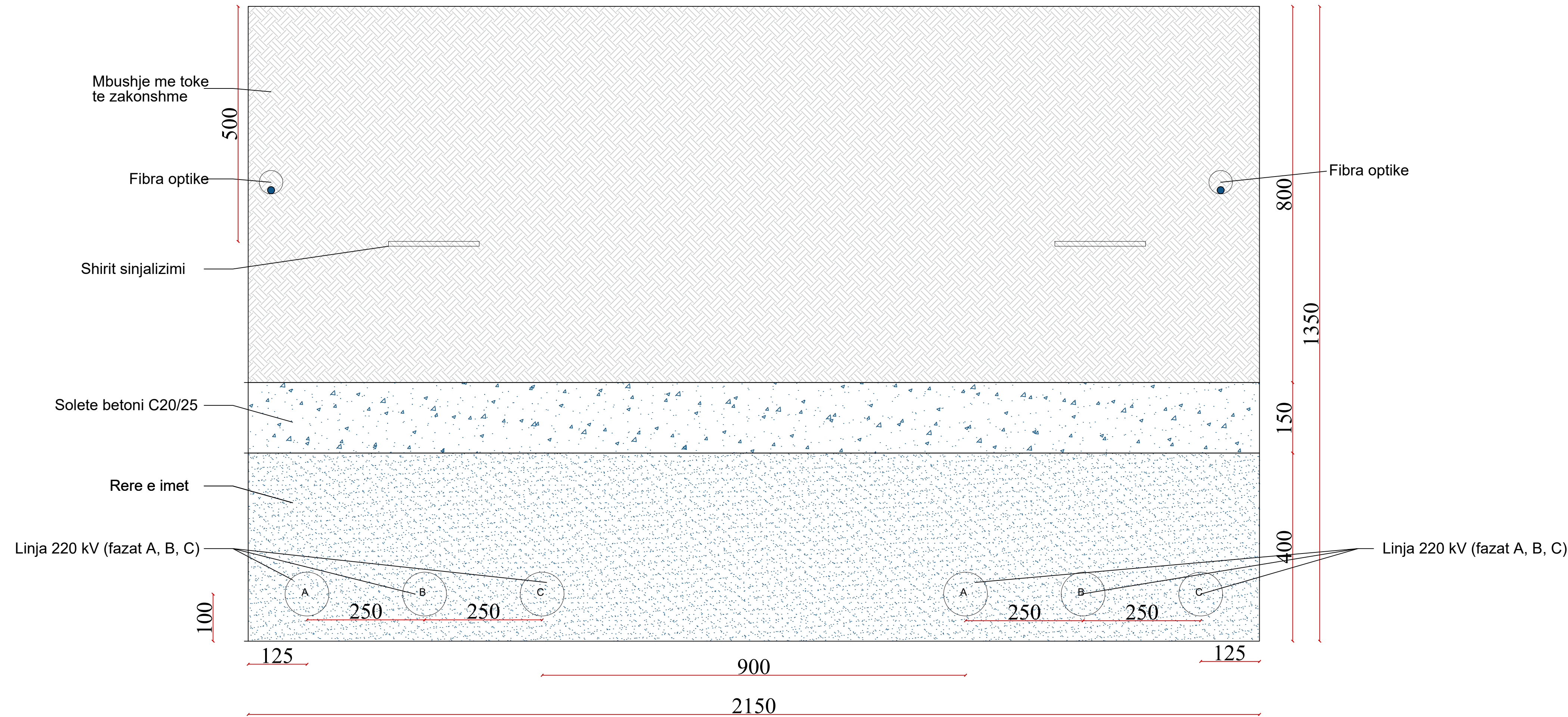
Tipi 1 (pa asfalt)
