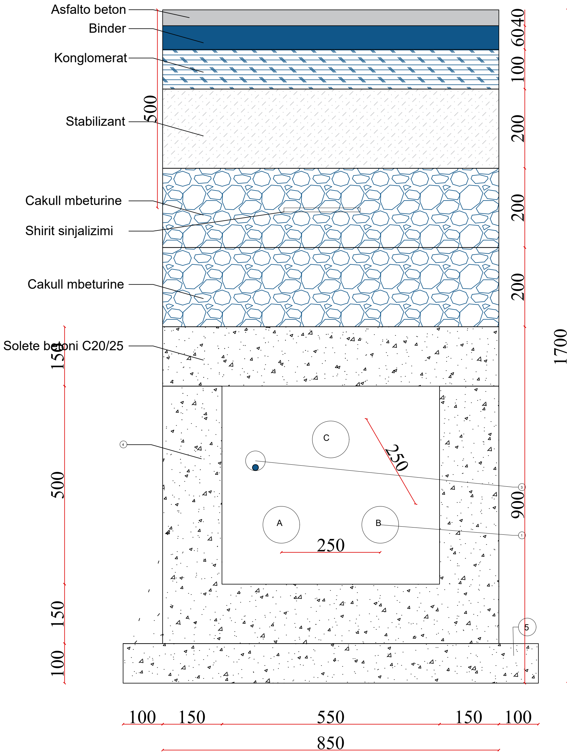
Tipi 2 me kanal betoni (me asfalt)
