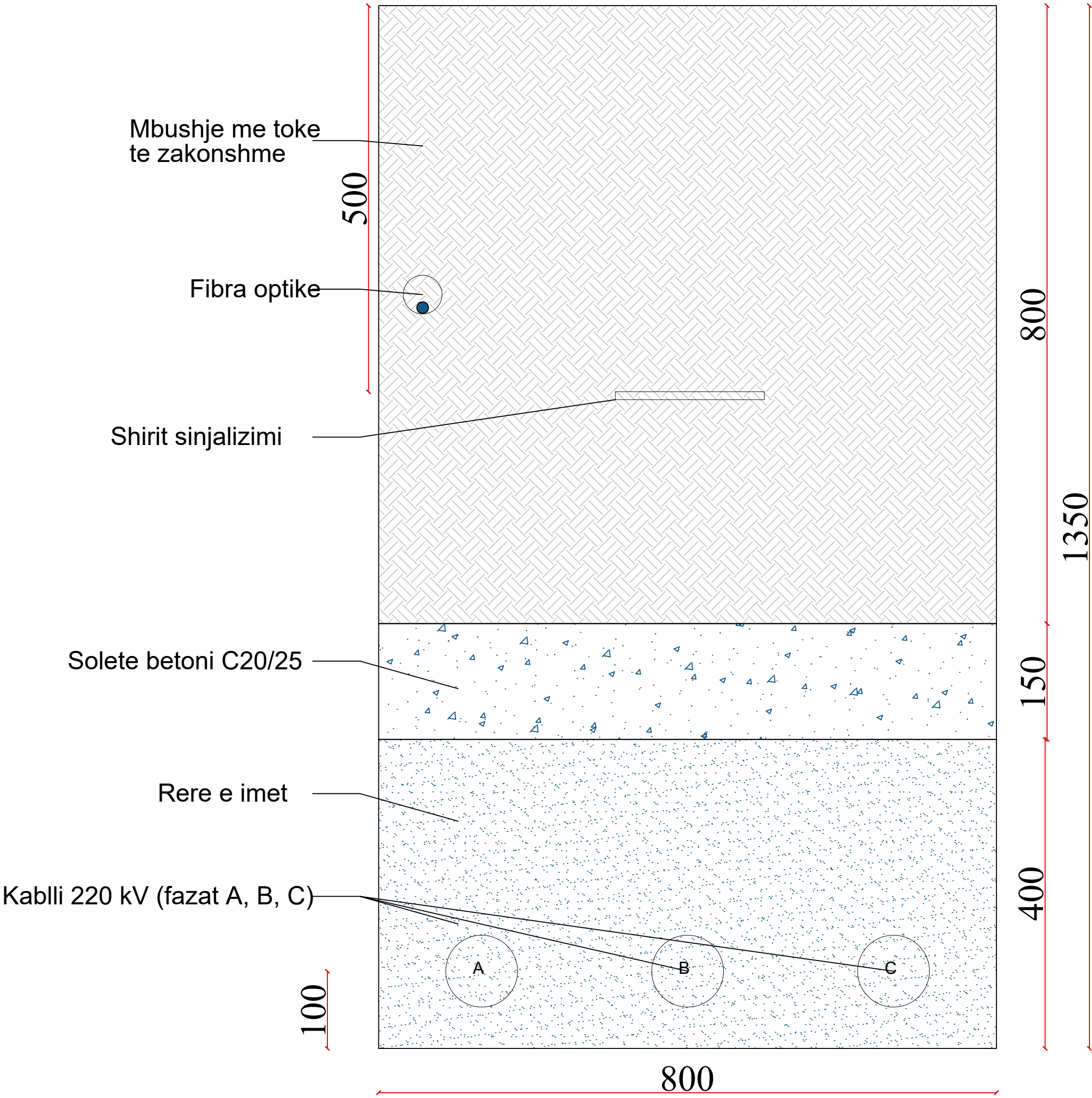
Tipi 1 (pa asfalt)
