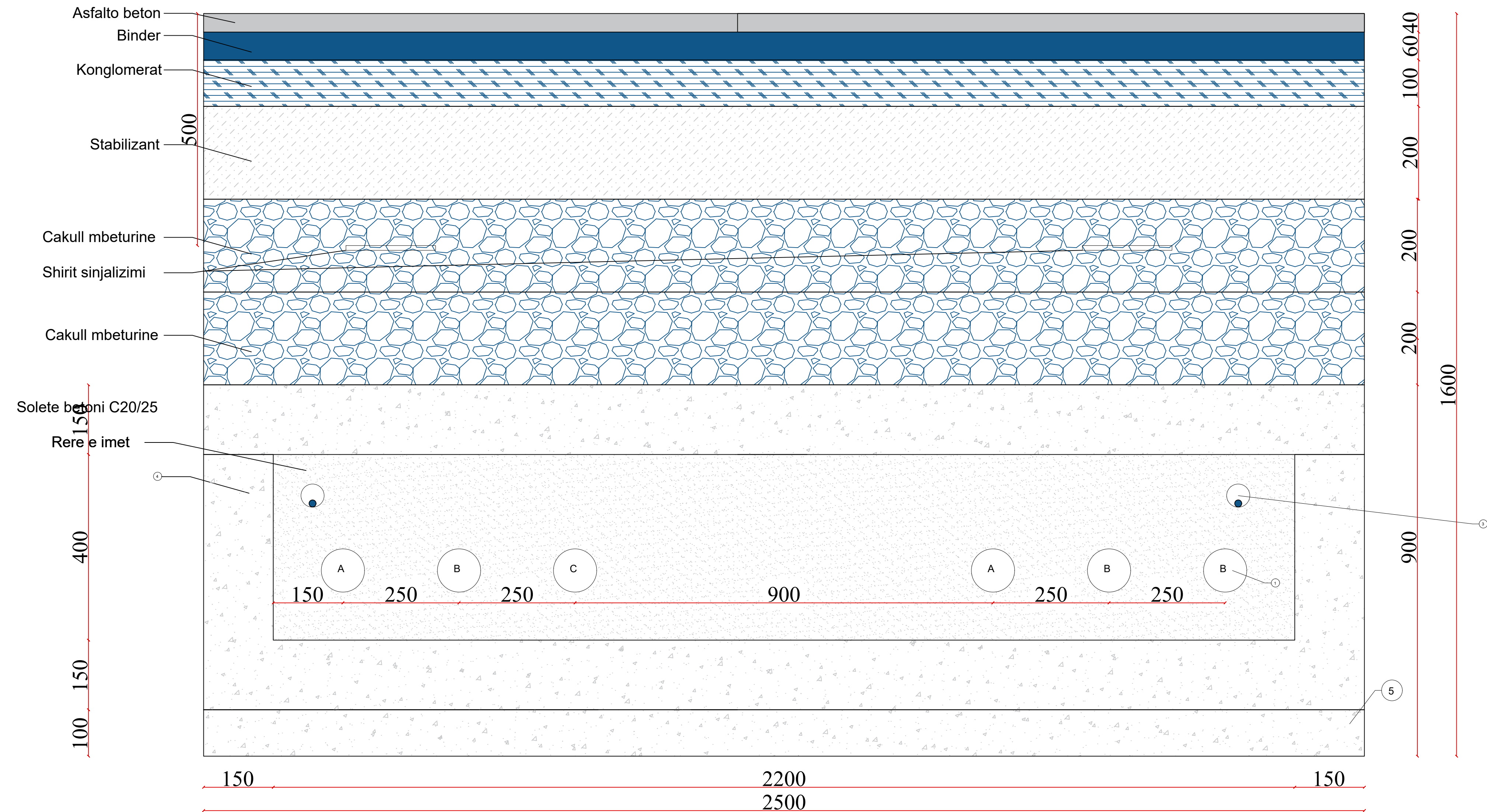
Tipi 2 me kanal betoni per dy qarqe linje (me asfalt)
