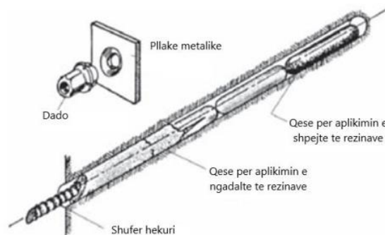
Figure I-9 - Elementet e Ankerave
