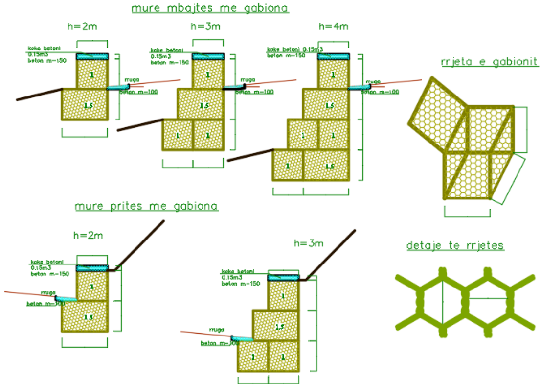
Figure II-9 - Detaje te murit mbajtese me gabiona
