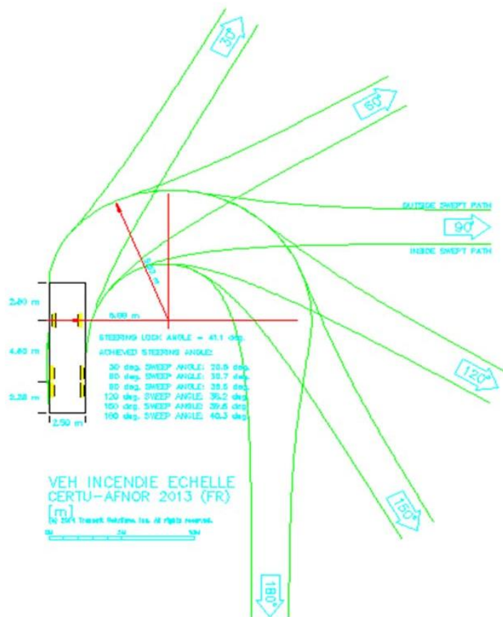
Figure II-8 - Te dhena teknike te mjetit te emergjences
