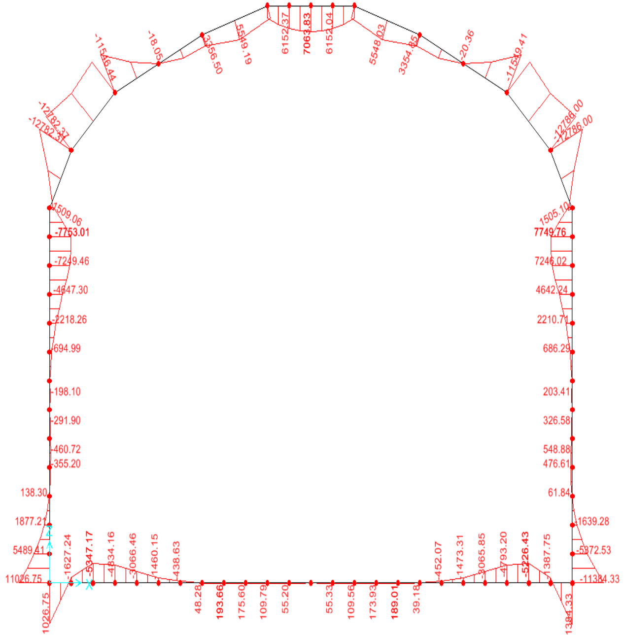
Figure I-14 - Epjura e momenteve
