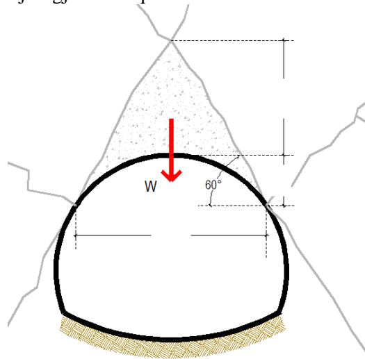
Figure I-11 - Skema teorike e punës së galerisë
