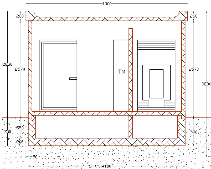
Prerja A-A
