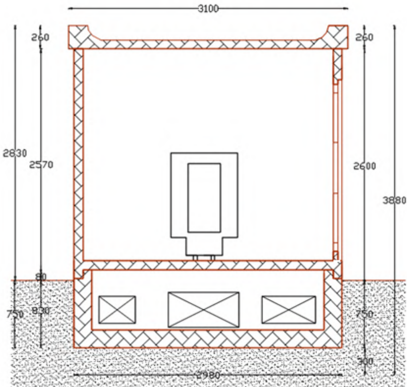
Prerja B-B
