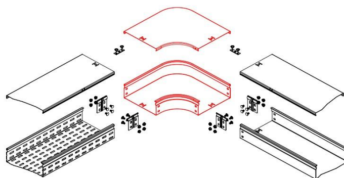
Figura 8-6Kanaline bashke me aksesoret
