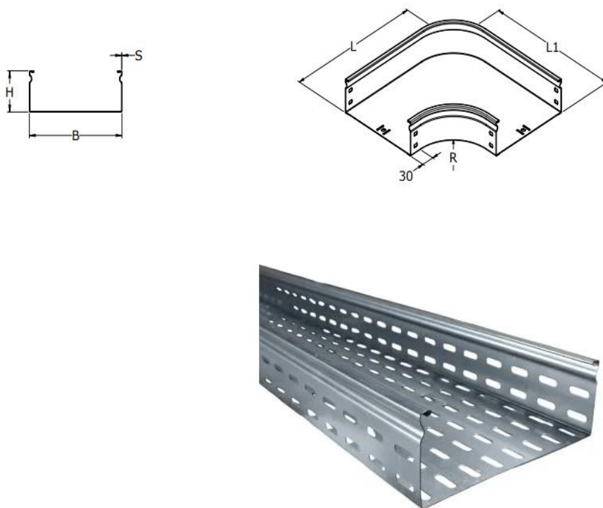
Figura 8-5: Paraqitje e detajeve te kanalinave
