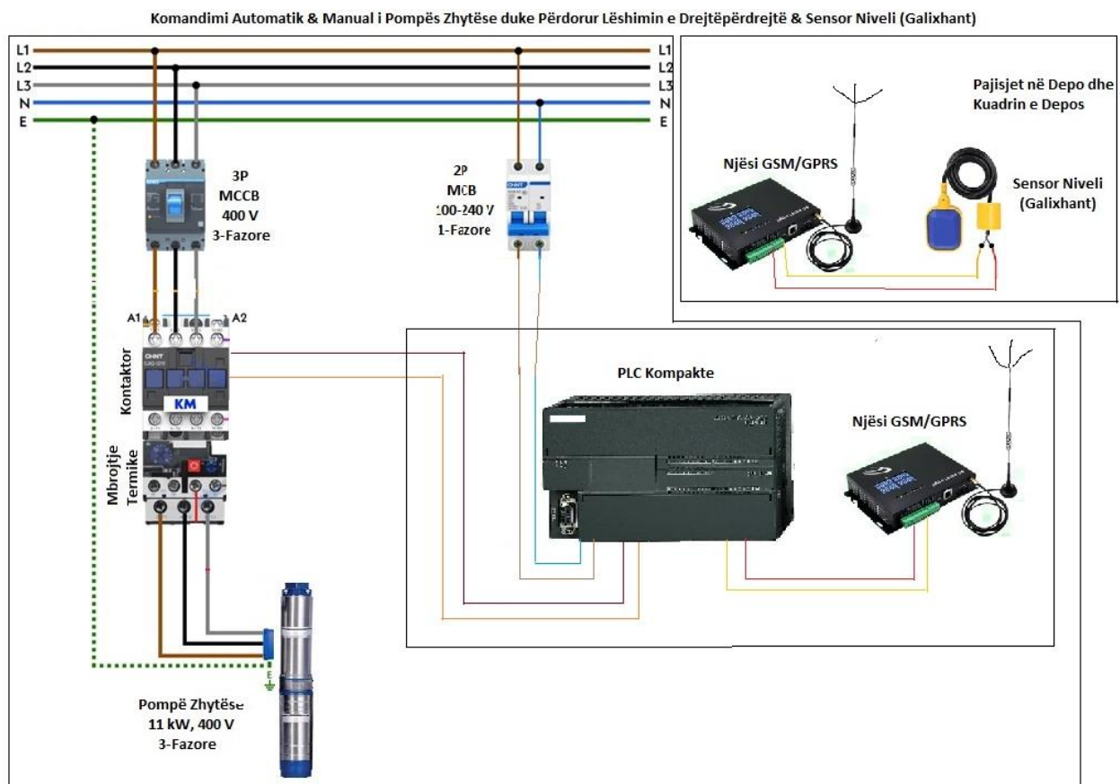
Figura 8-10: Skema e komandimit të pompës zhytëse dhe nivelit të ujit të deposë re nëpërmjet sistemit PLC-SCADA
