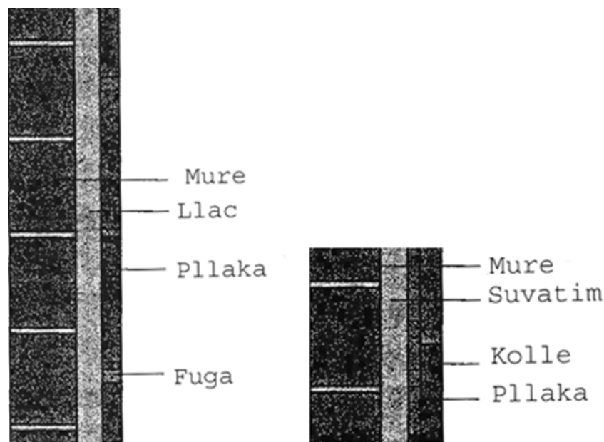
Figura 10-1: paraqitje skematike e vendosjes së pllakave në mure
