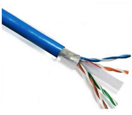
Figura 8-9: Kablo CAT 6 FTP
