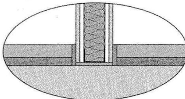
Figura 9-2: detaj i hollesishem i lidhjes se murit te gipsit ne prerjen vertikale
