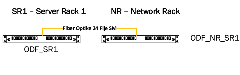
Figure 9 - Diagrama e Lidhjes se ODF-ve
