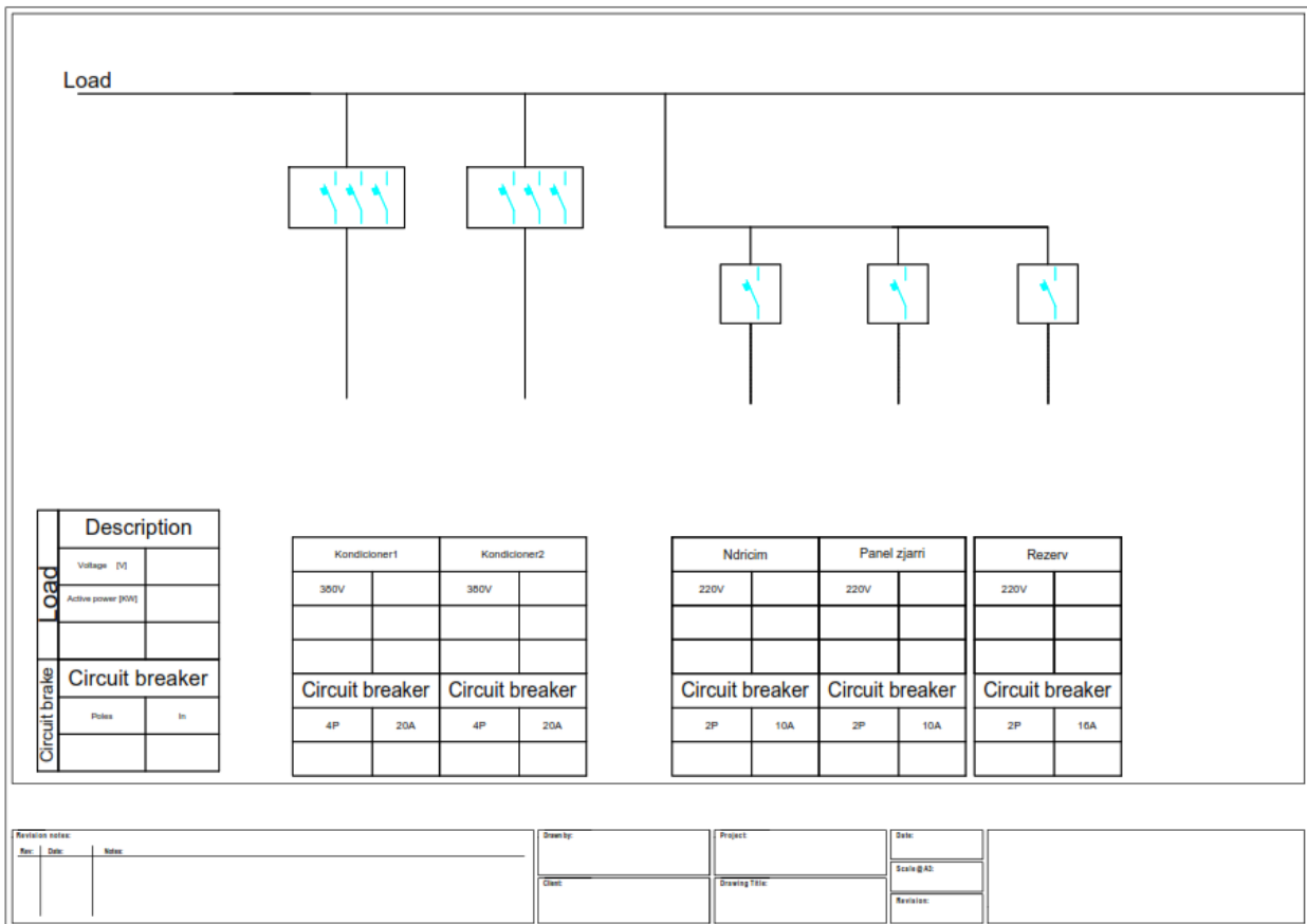
Figure 6 - Skema e panelit per furnizimin e AC dhe sistemeve te tjera (ilustrim)
