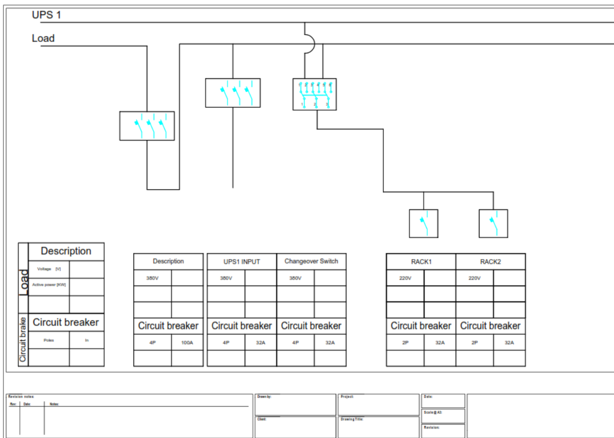
Figure 4 - Skema e Panelit per furnizimin nga UPS_1 (ilustrim)
