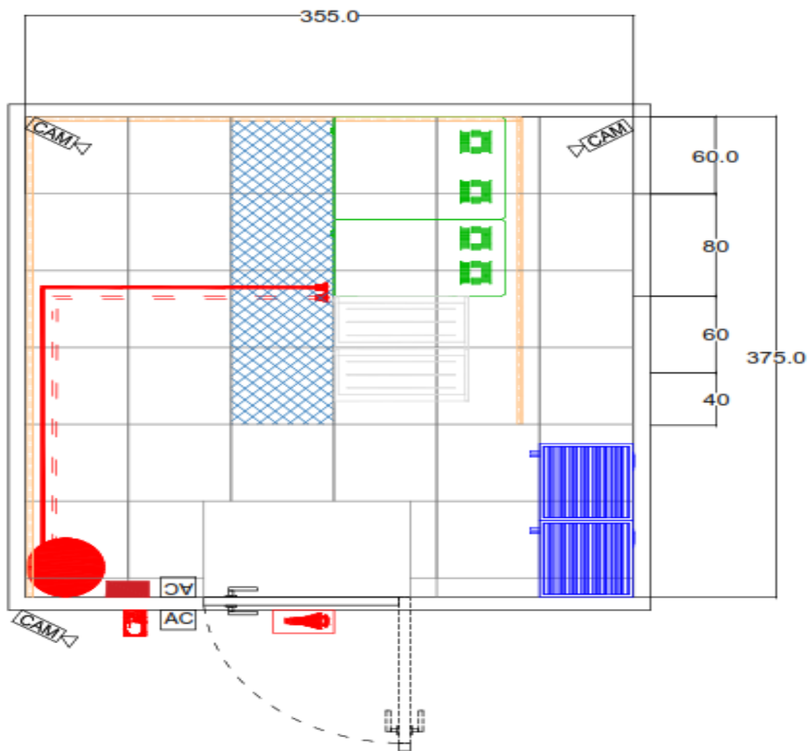
Figure 1 - Planvendosja e Paisjeve ne Dhome
