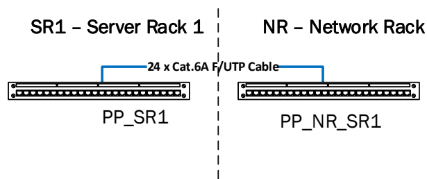
Figure 10 - Diagrama e Lidhjes se Patch Paneleve
