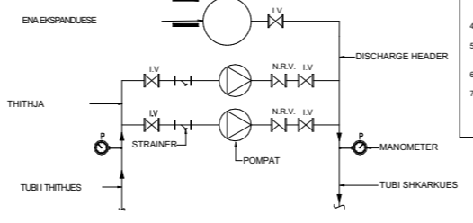
6 DETAL TIPIK PER SETIN E POMPAVE SANITARE WS-01
