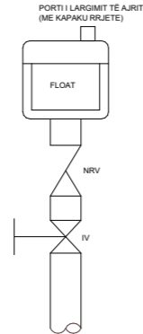
2 DETAL TIPIK TË VALVULES AUTOMATIKE TË AJRIT (AAV) WS-01
