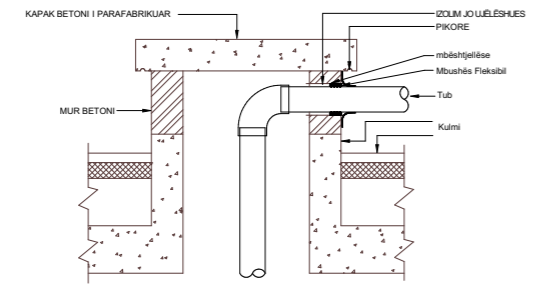
5 Tubat tipik në penthouse WS-01
