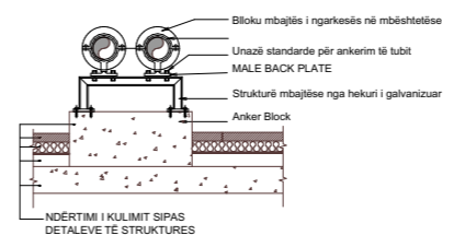
4 MBËSHTETJA STANDARDE - TUBAT NË KULM WS-01
