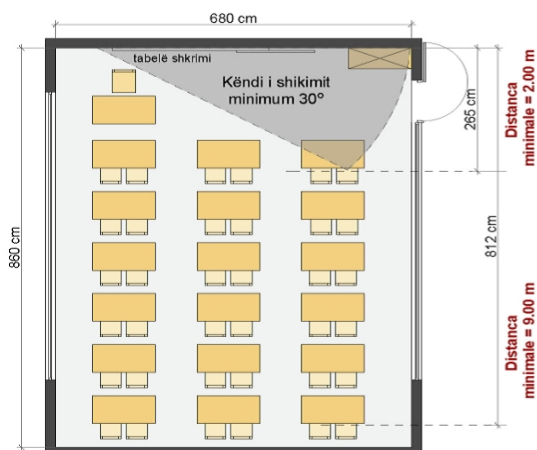
KOMODITETI PËR DHOMË MËSIMI ME 3 RENDE BANKASH (30-36 dhe 42 nxënës në raste të jashtëzakonshme)
