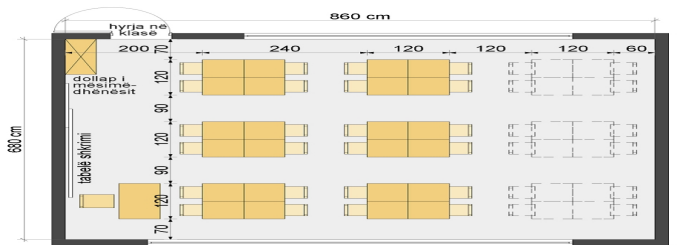
Mësimi në grupe Organizimi i dhomës së mësimi me një tavolinë për një nxënës Niveli I Mësim, 24 ose 36 nxënës, Orenditë e kategorisë "C"
