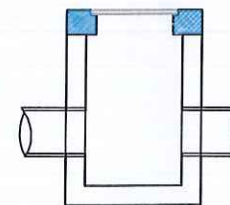
SEKSIONI 1-1 SH 1:50
