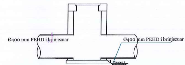
SEKSIONI 1-1 SH 1:50
