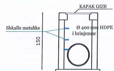
SEKSIONI 2-2 SH 1:50
