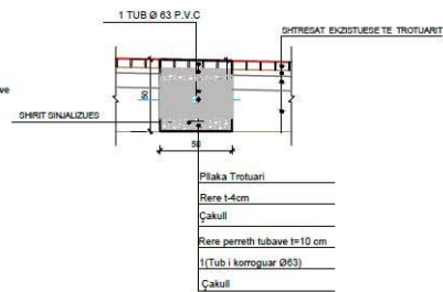
Paketa e shtresave në trotuar
