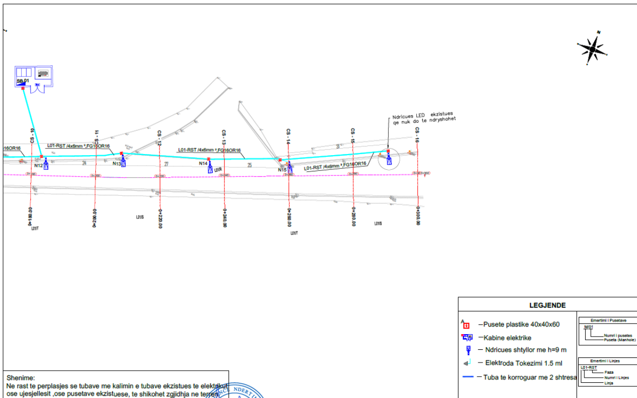
Figura 3: Planimetria e ndrcimit rruga “Wilson” dhe sheshit “2 Prilli”
