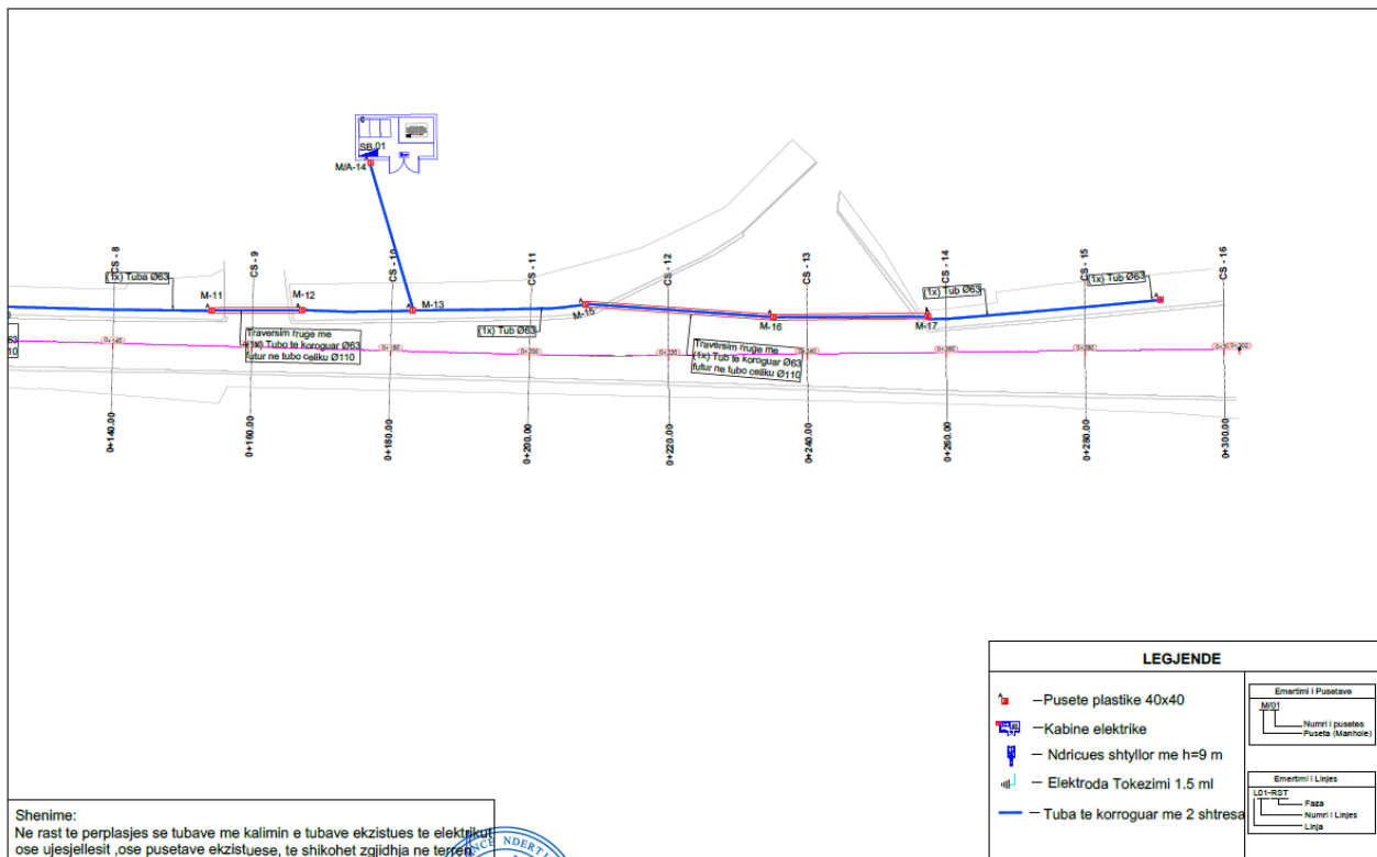
Figura 4: Planimetria e linjave te ndricimit rruga “Wilson” dhe sheshit “2 Prilli”
