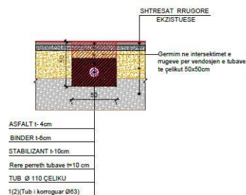
Prerje terhorë e tubacionit në rrugë
