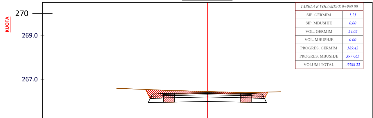
CS - 49 PROG - 0+960.0
