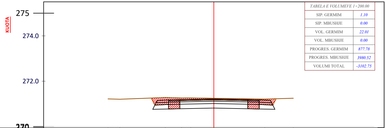
CS - 61 PROG - 1+200.0
