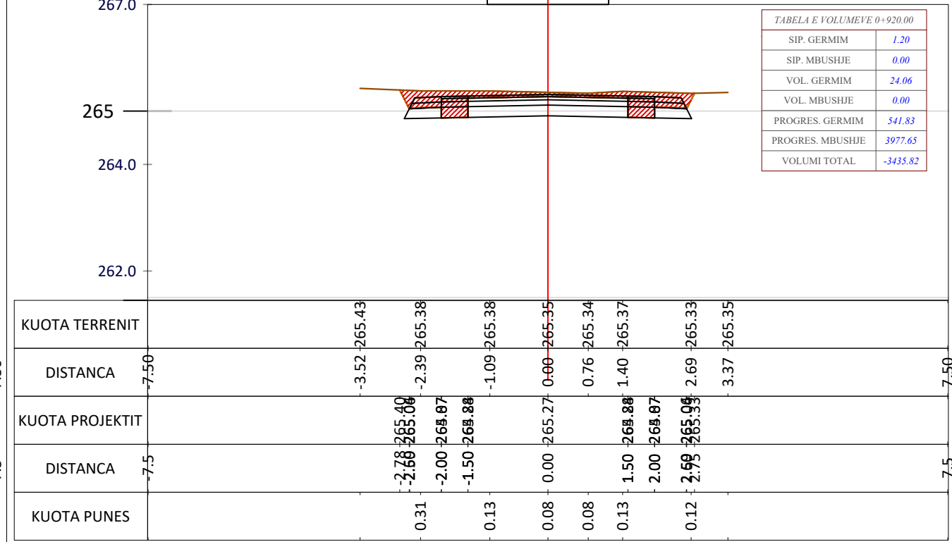
CS - 47 PROG - 0+920.0
