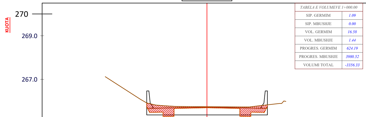
CS - 51 PROG - 1+000.0
