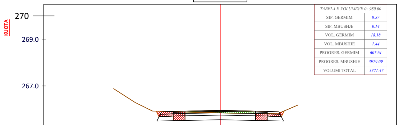
CS - 50 PROG - 0+980.0
