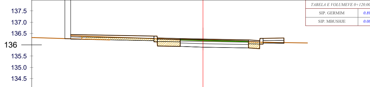
CS - 7 PROG - 0+120.0
