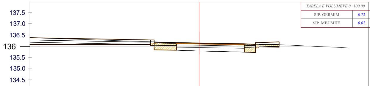
CS - 6 PROG - 0+100.0
