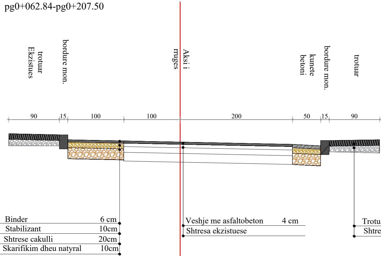
PROFILI TIP 1:40
