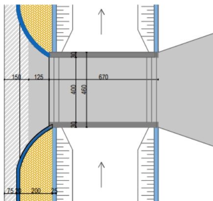
PLANIMETRI URA SHK. 1 :100
