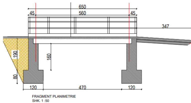
SEKSIONI TERTHOR URA SHK. 1 :50
